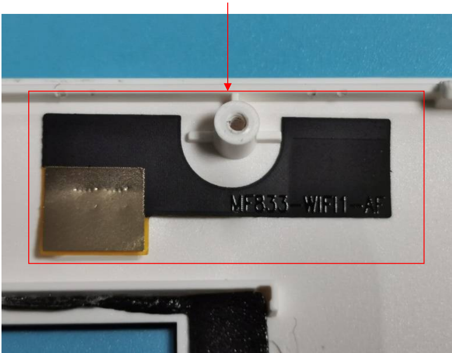
Wi-Fi ANT1
