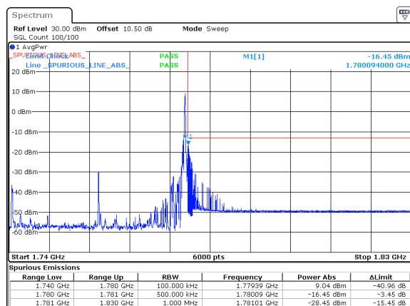
n66_40MHz_15kHz_1760MHz_DFT-s-OFDM QPSK_RB1@215
