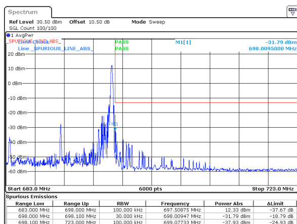
n71_15MHz_15kHz_690.5MHz_DFT-s-OFDM QPSK_RB1@78
