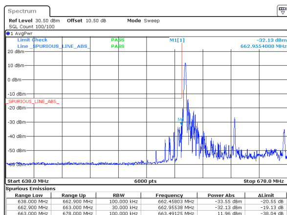
n71_15MHz_15kHz_670.5MHz_DFT-s-OFDM QPSK_RB1@0
