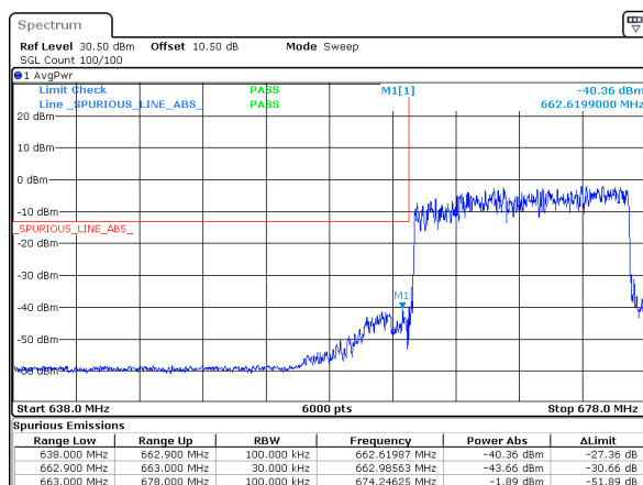
n71_15MHz_15kHz_670.5MHz_DFT-s-OFDM QPSK_RB75@0
