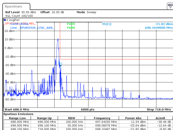
n71_10MHz_15kHz_693MHz_DFT-s-OFDM QPSK_RB1@51
