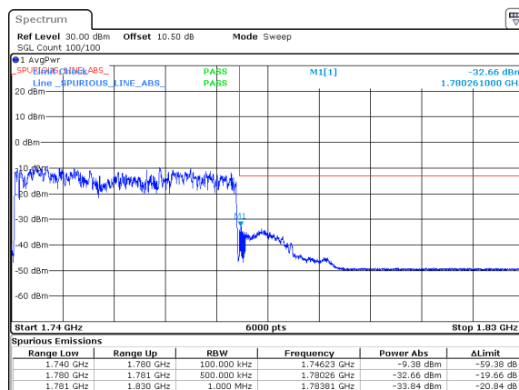
n66_40MHz_15kHz_1760MHz_DFT-s-OFDM QPSK_RB216@0
