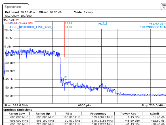
n71_15MHz_15kHz_690.5MHz_DFT-s-OFDM QPSK_RB75@0
