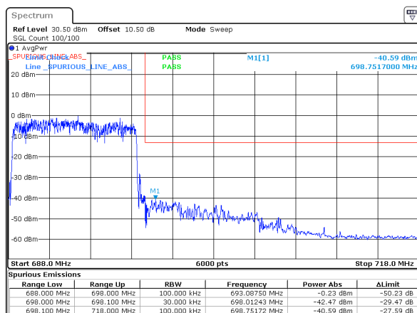
n71_10MHz_15kHz_693MHz_DFT-s-OFDM QPSK_RB50@0
