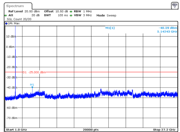
20MHz_Low_QPSK_1@0(1GHz~27.2GHz)
