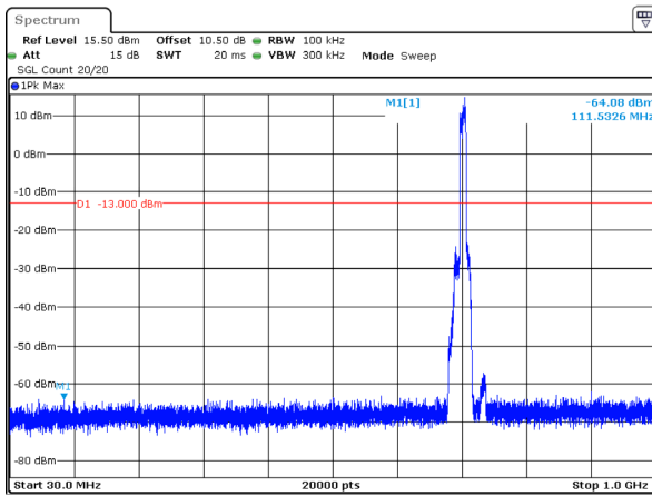
10MHz_Middle_QPSK_50@0(30MHz~1GHz)
