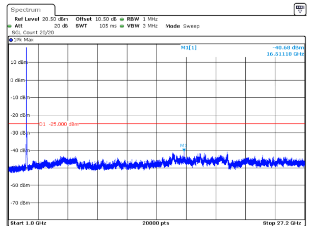
20MHz_Low_QPSK_100@0(1GHz~27.2GHz)
