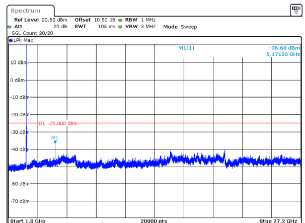
20MHz_Middle_QPSK_1@0(1GHz~27.2GHz)
