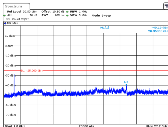
10MHz_Middle_QPSK_50@0(1GHz~27.2GHz)
