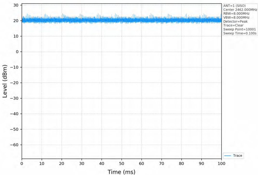
802.11n(HT20)_2462.000MHz_SISO_ANT1
