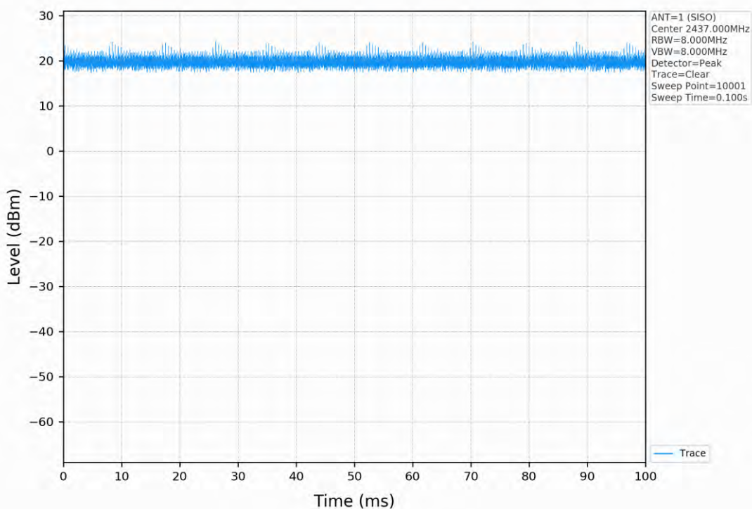
802.11g_2437.000MHz_SISO_ANT1
