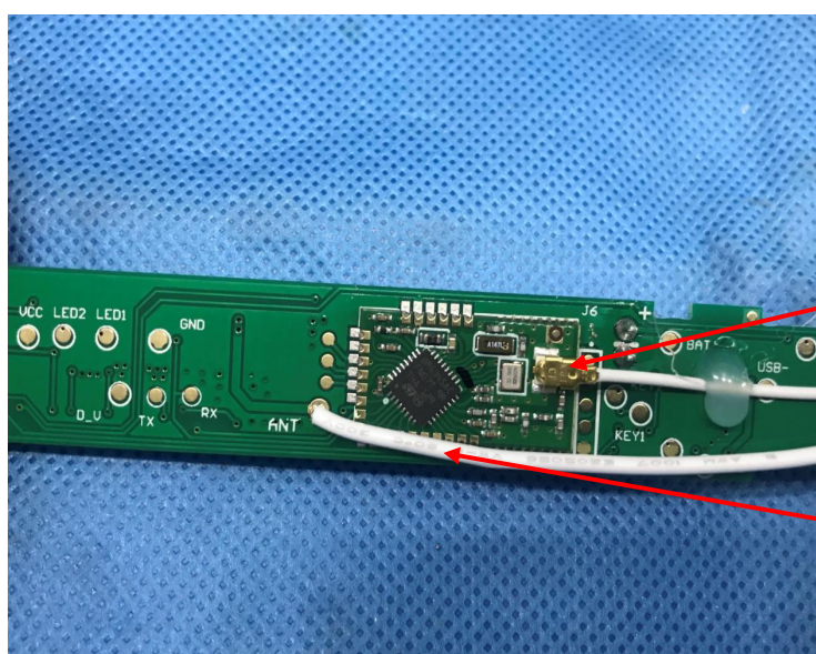
BLE module
