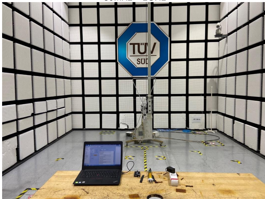
30MHz ~ 1GHz
