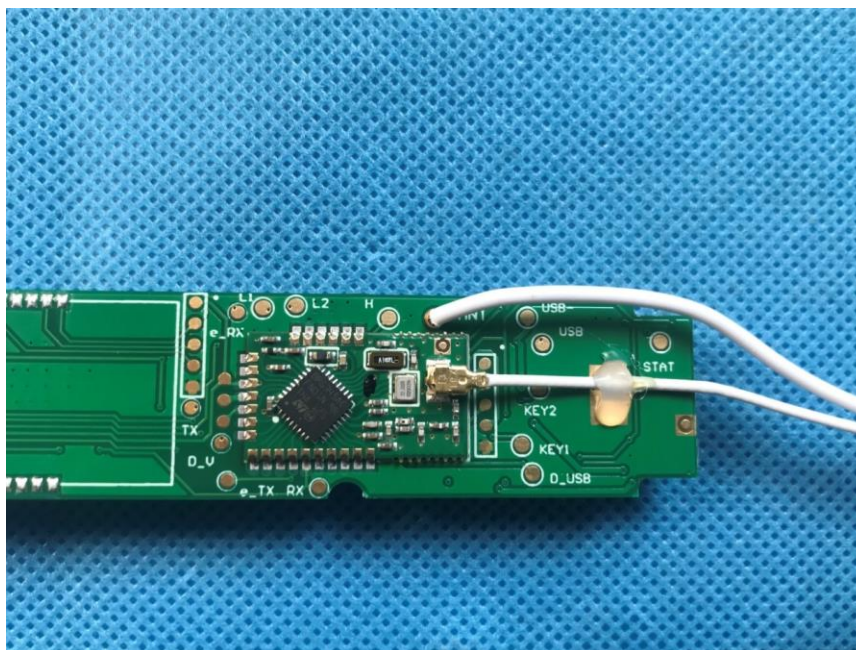
BLE module
