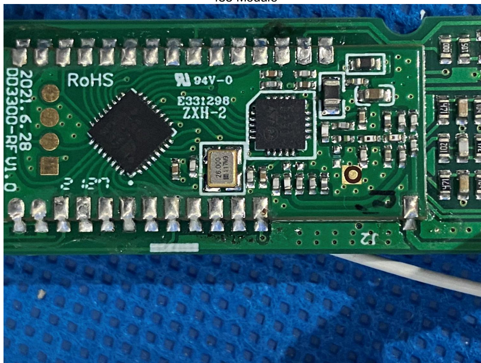
433 Module
