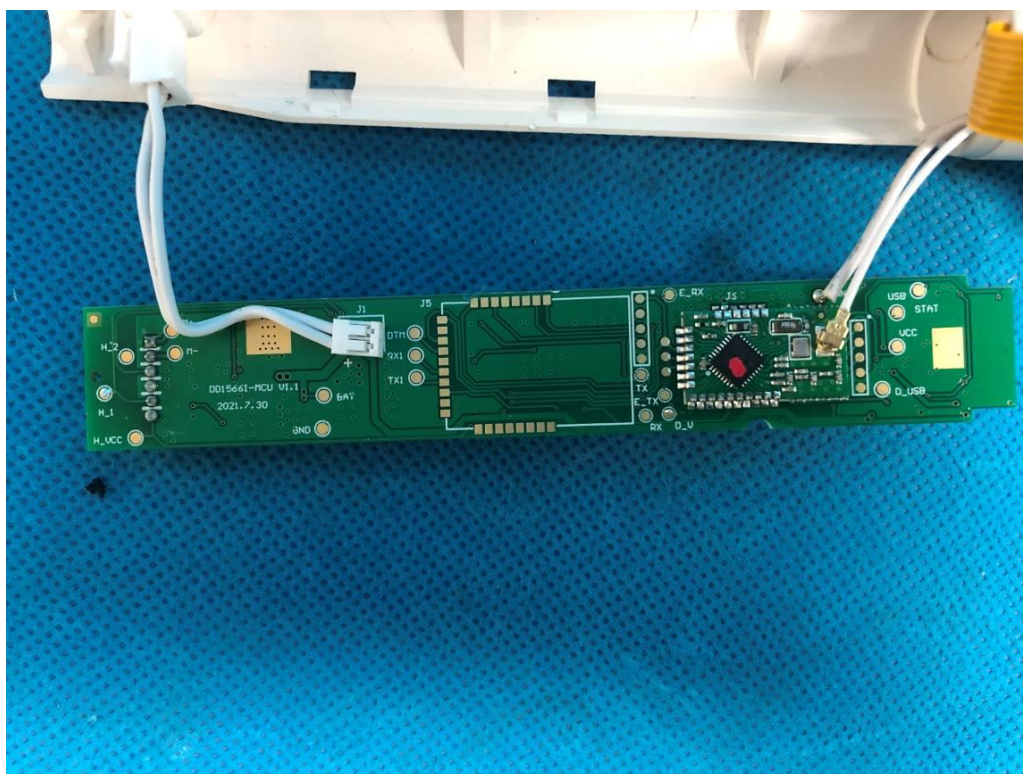
433 Module
