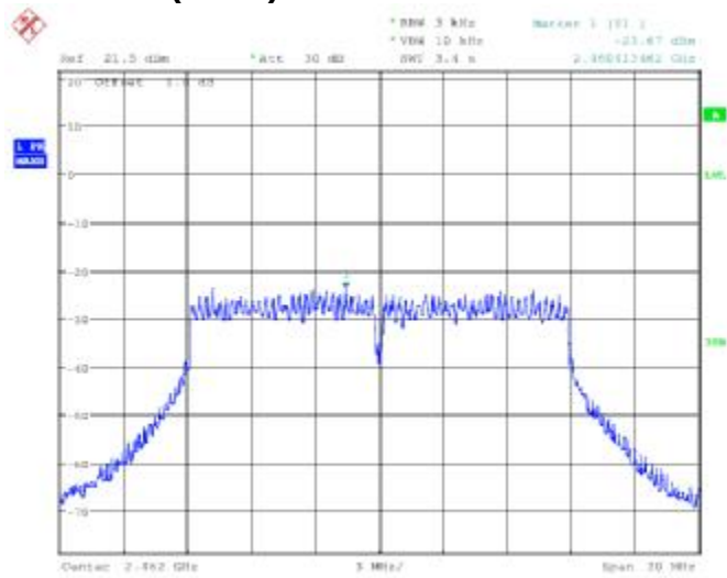
802.11n(HT20) 2462MHz
