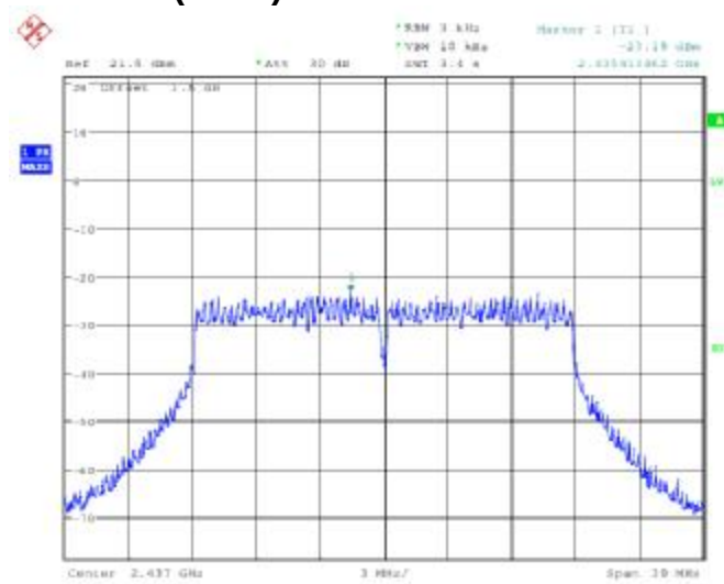
802.11n(HT20) 2437MHz
