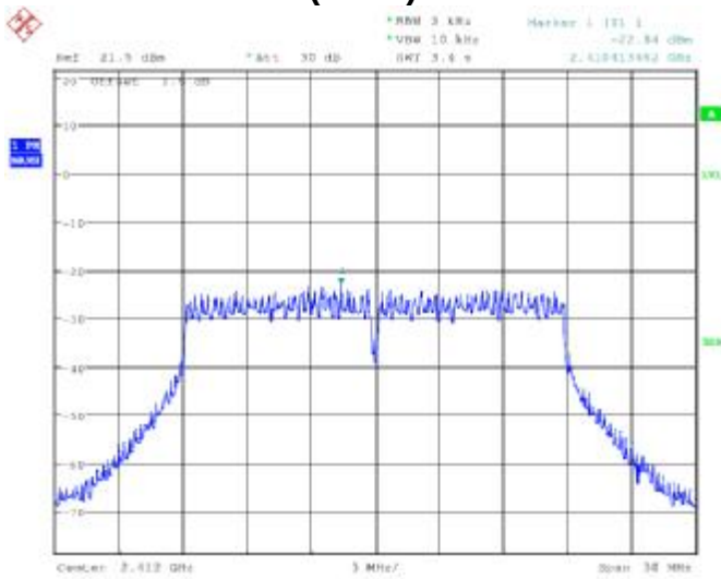
802.11n(HT20) 2412MHz
