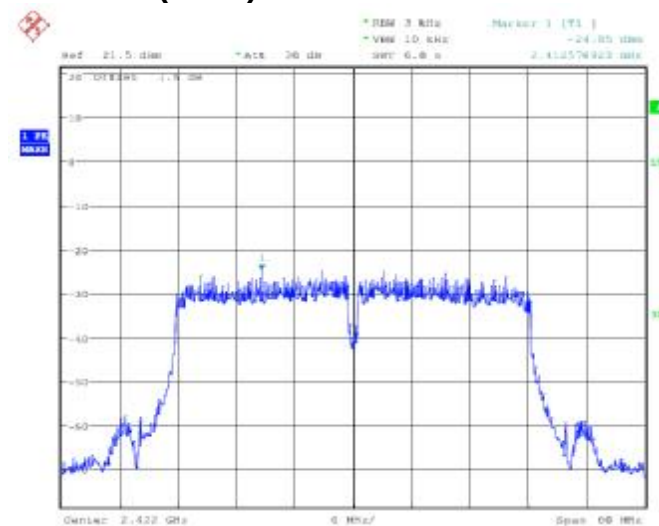
802.11n(HT40) 2422MHz
