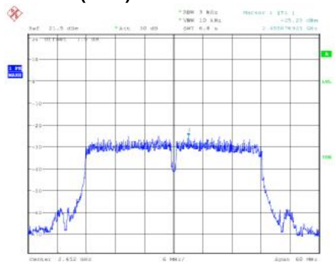
802.11n(HT40) 2452MHz
