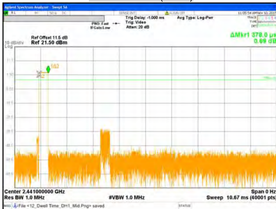
DH1 CH Middle (GFSK)
