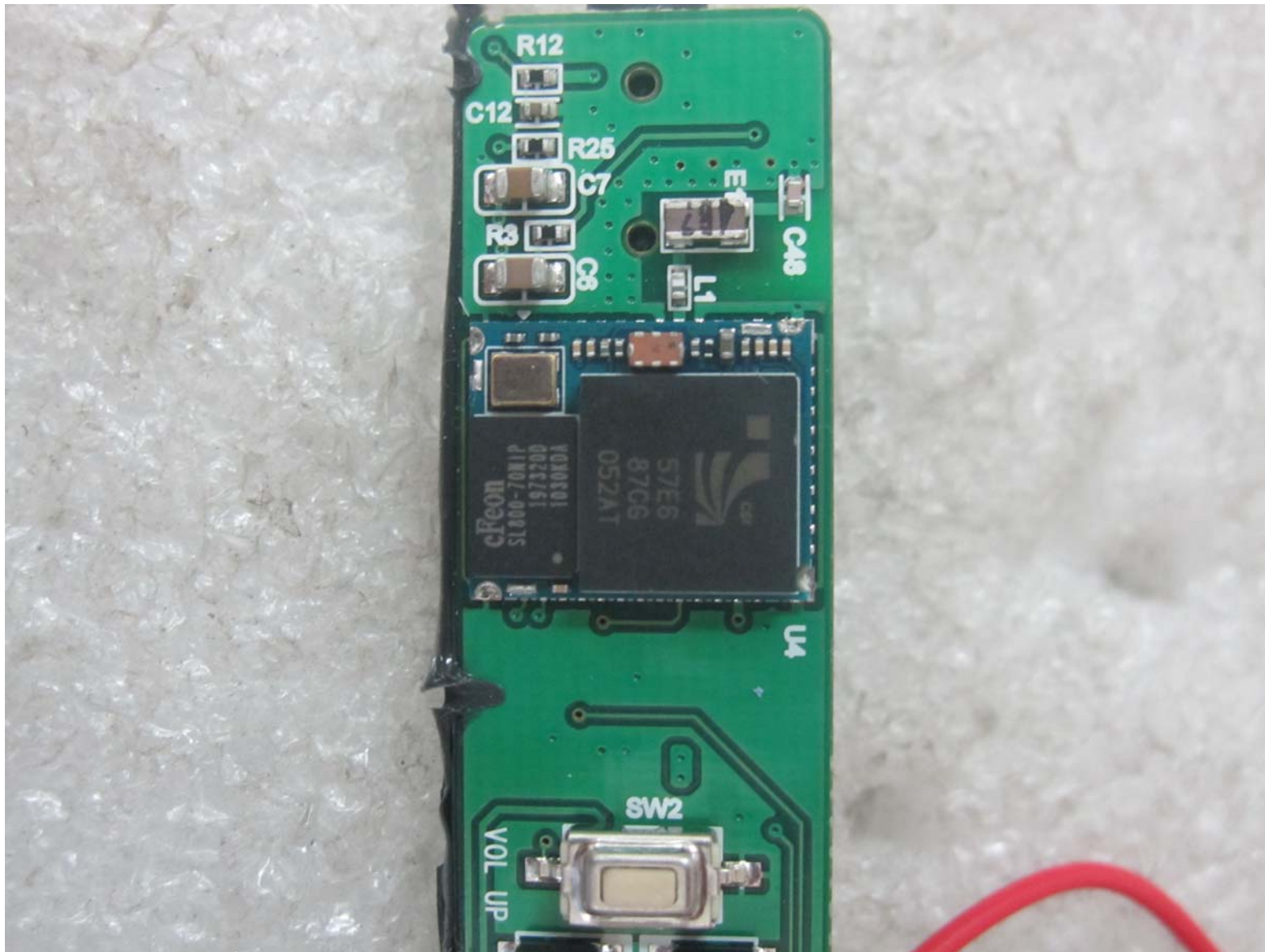
EXB100_RF Module
