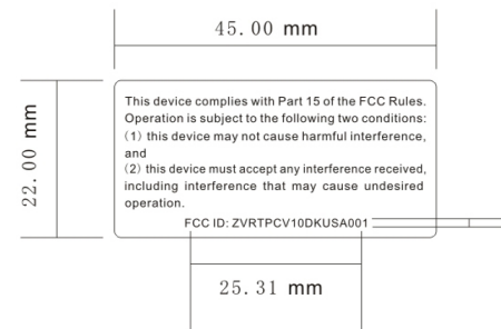
贴纸1:1视图，边框不丝印
