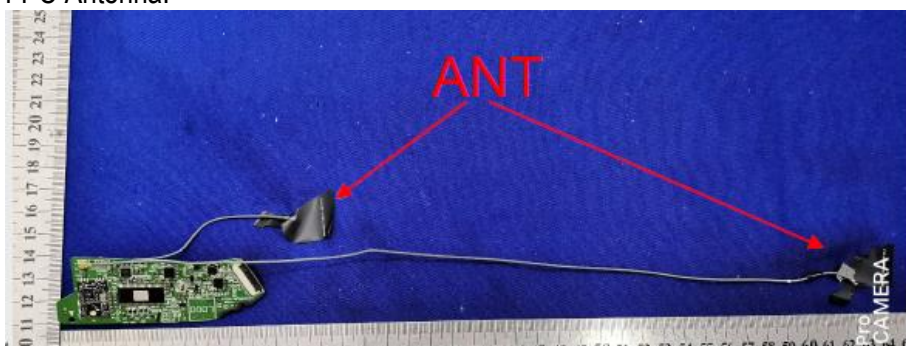
FPC Antenna:
