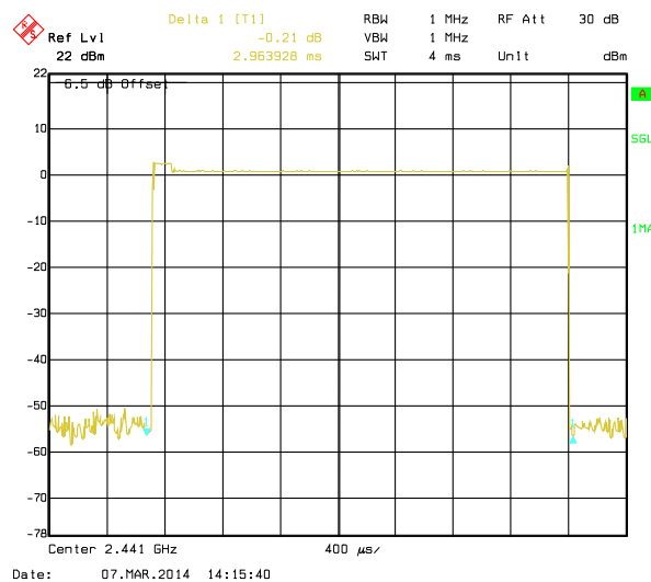
2-DH5
