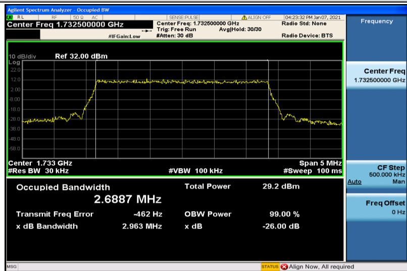
Band4-3MHz-QPSK-20175-15RB#0-2.6887
