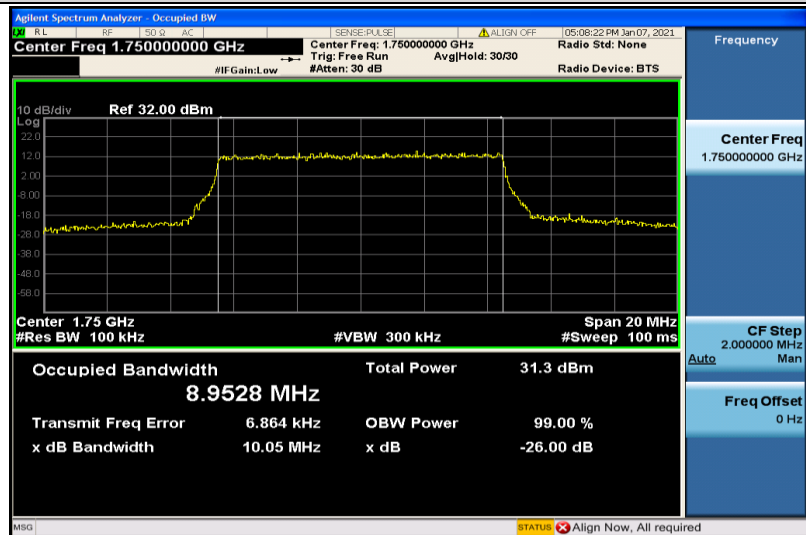
Band4-10MHz-QPSK-20350-50RB#0-8.9528
