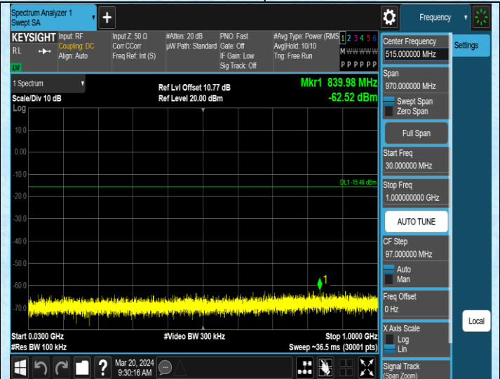
11G-Ant1-2437-30~1000-PASS
