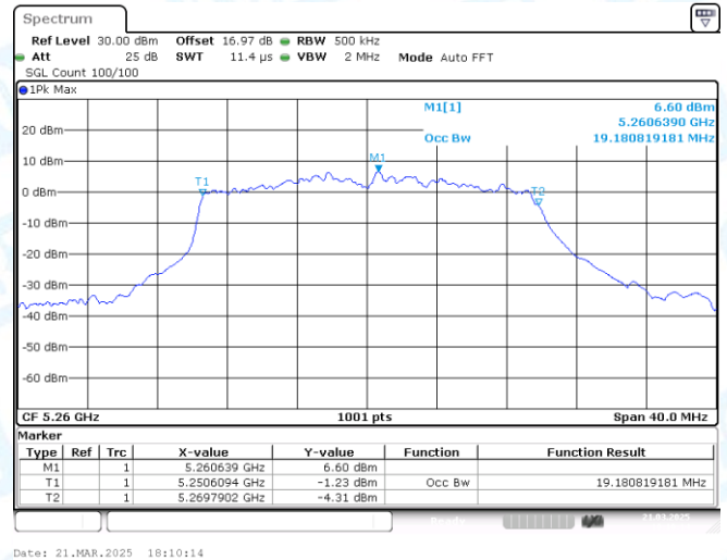
11AX20MIMO-Ant1-5260
