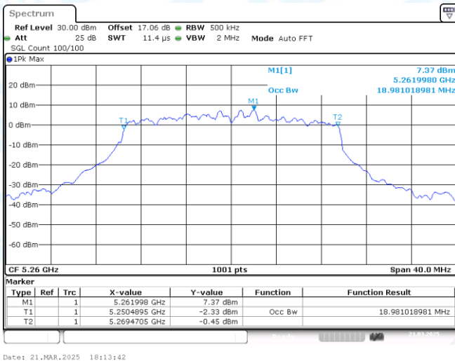
11AX20MIMO-Ant2-5260
