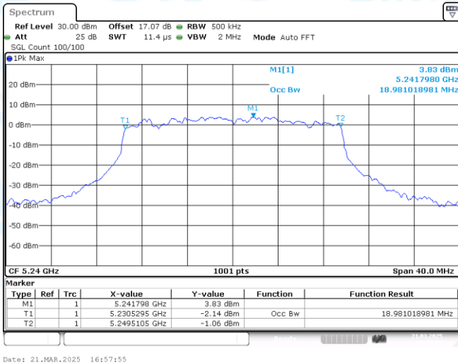
11AX20MIMO-Ant2-5240
