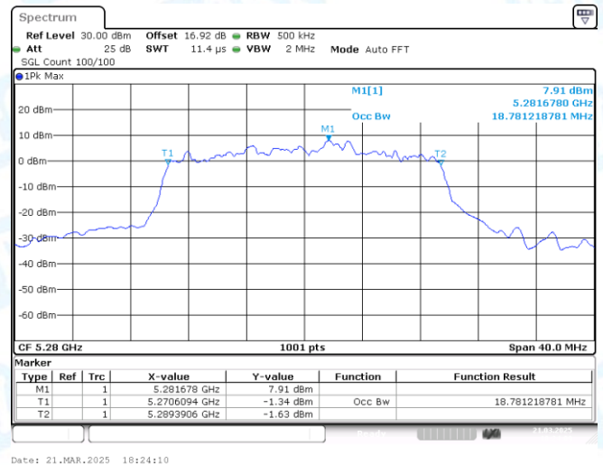
11AX20MIMO-Ant1-5280
