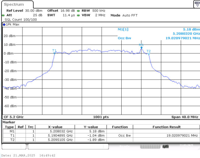
11AX20MIMO-Ant2-5200
