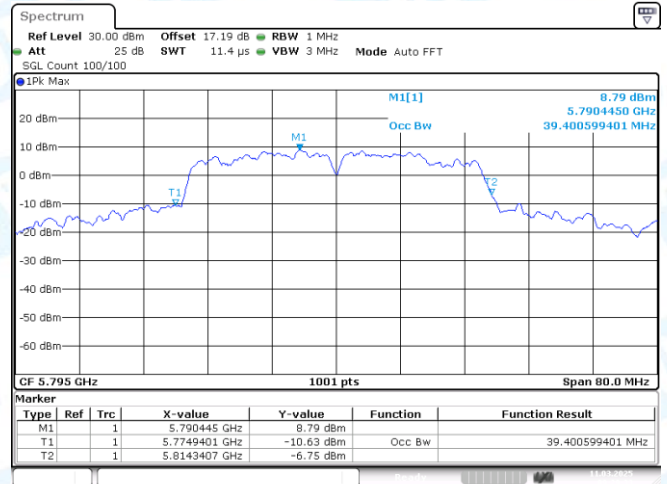
11AC40MIMO-Ant1-5795
