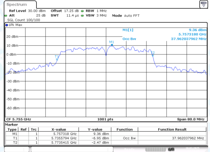
11N40MIMO-Ant1-5755
