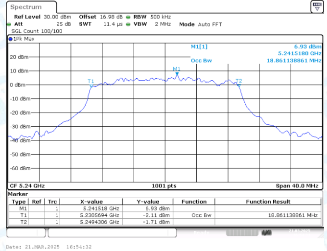
11AX20MIMO-Ant1-5240
