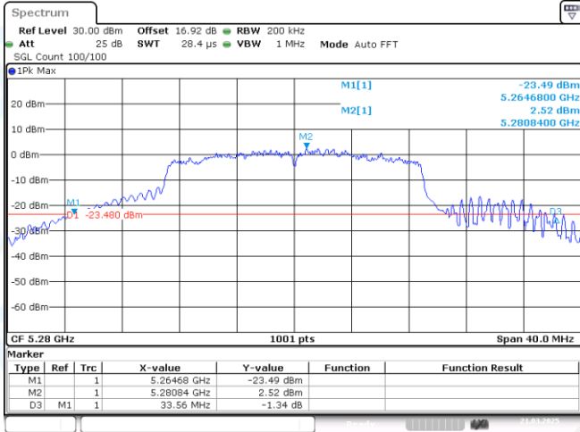
11AC20MIMO-Ant1-5280
