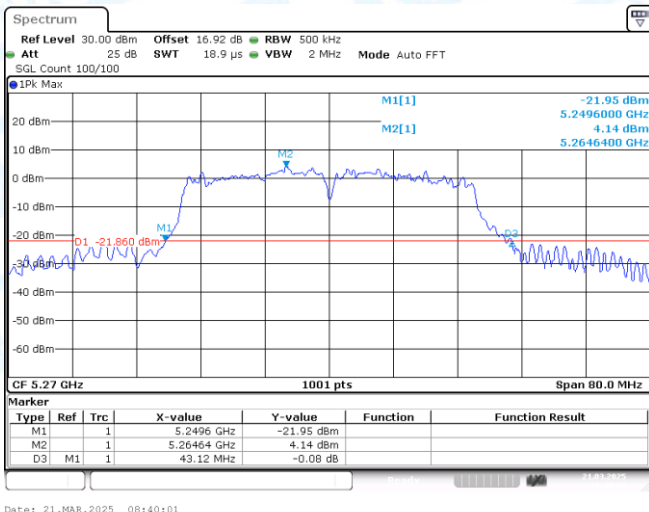
11N40MIMO-Ant1-5270
