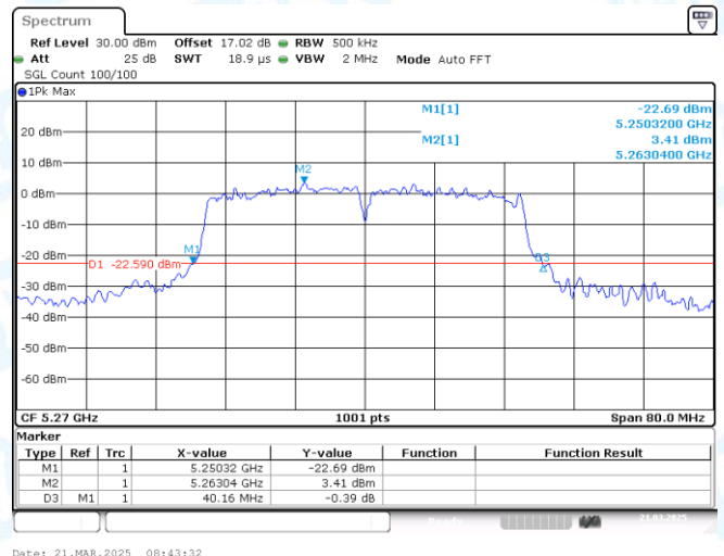
11N40MIMO-Ant2-5270
