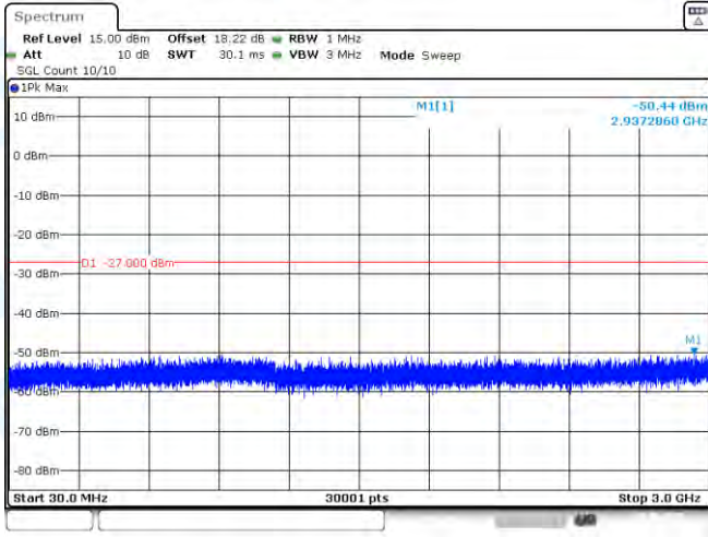
11AX80SISO-Ant1-6545-30~3000-PASS
