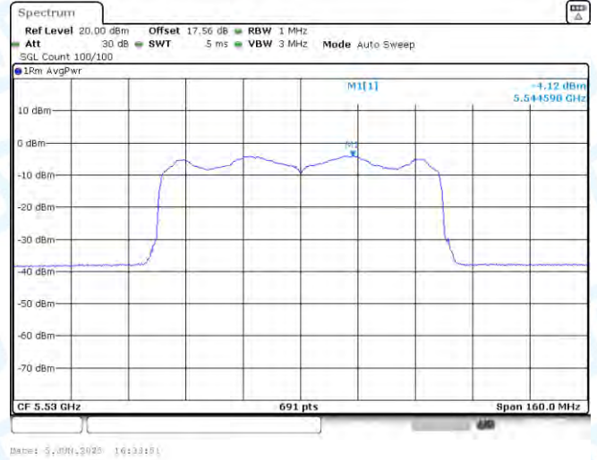
11AX80SISO-Ant1-5530-PASS
