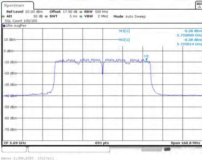
11AC80SISO-Ant1-5690_UNII-3-PASS
