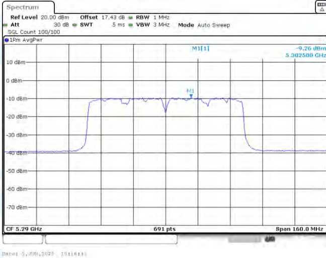
11AC80SISO-Ant1-5290-PASS
