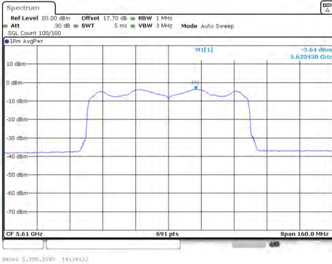
11AX80SISO-Ant1-5610-PASS
