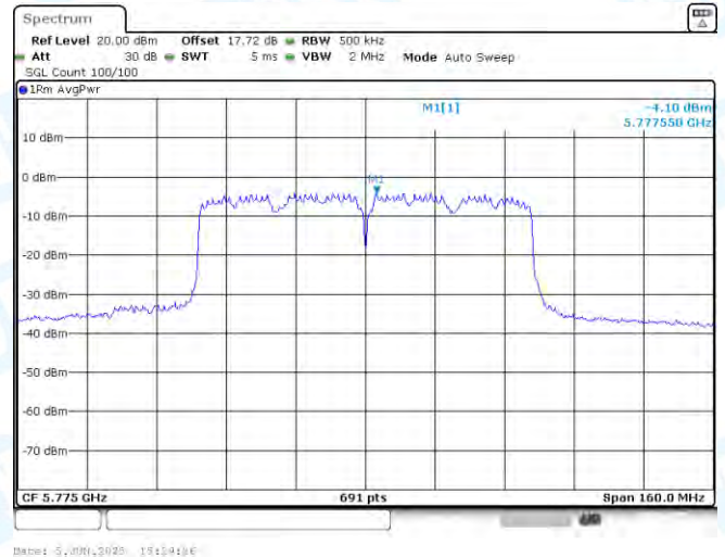
11AC80SISO-Ant1-5775-PASS
