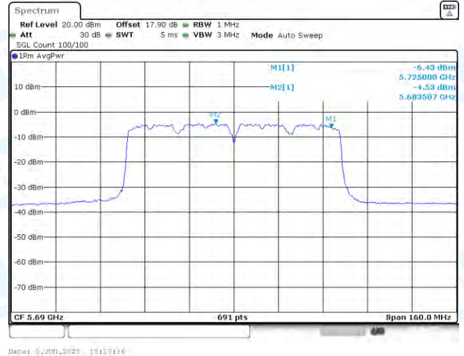
11AC80SISO-Ant1-5690_UNII-2C-PASS
