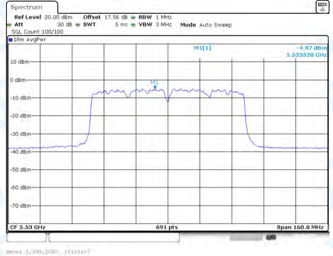
11AC80SISO-Ant1-5530-PASS
