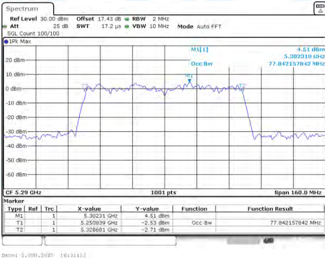
11AX80SISO-Ant1-5290
