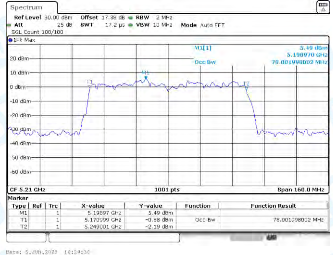
11AX80SISO-Ant1-5210
