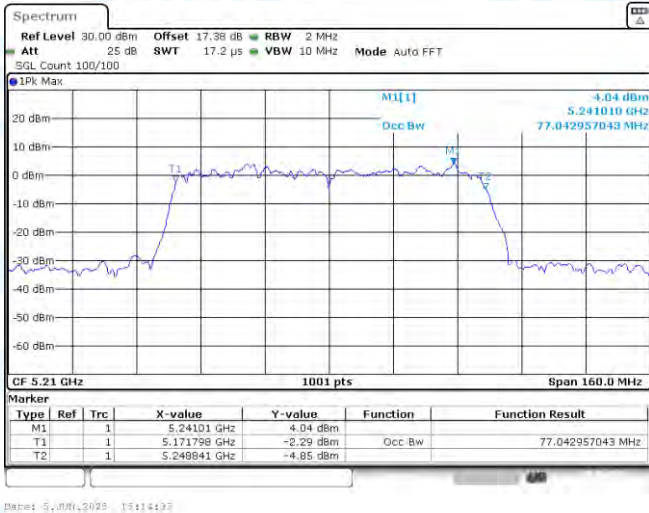
11AC80SISO-Ant1-5210
