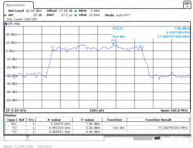
11AX80SISO-Ant1-5530
