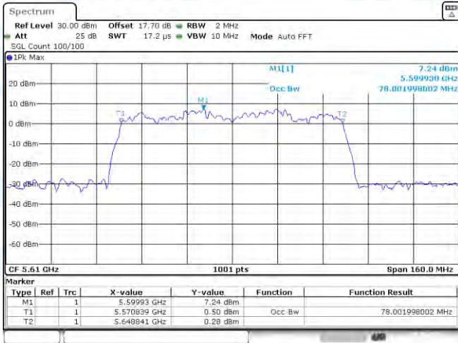
11AX80SISO-Ant1-5610
