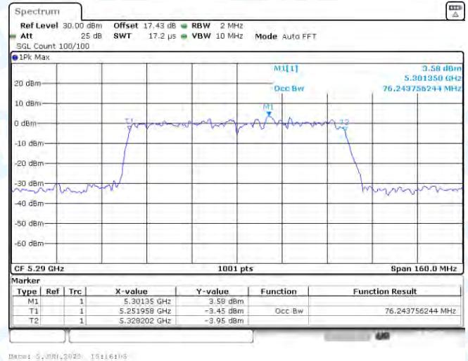
11AC80SISO-Ant1-5290
