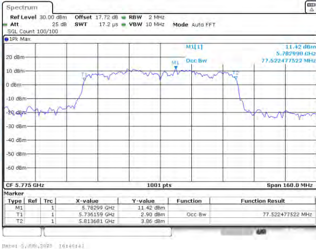
11AX80SISO-Ant1-5775
