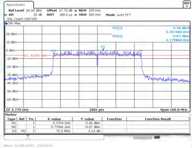
11AC80SISO-Ant1-5775-PASS
