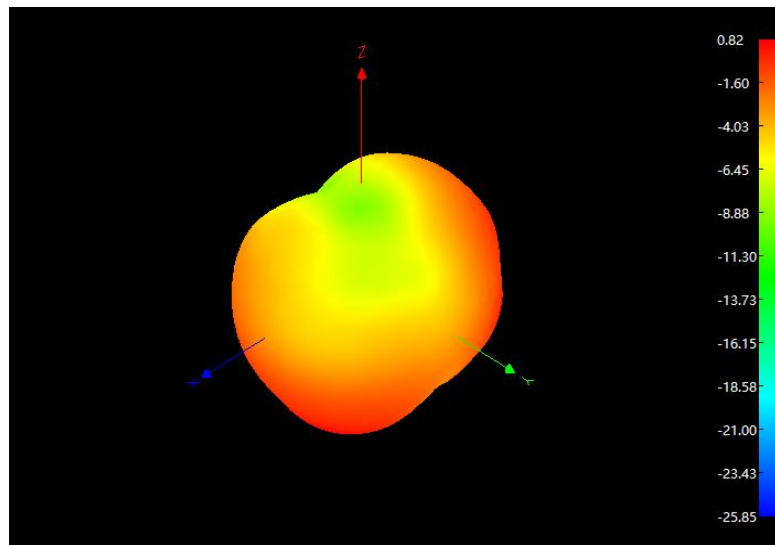
2450MHz 3D
