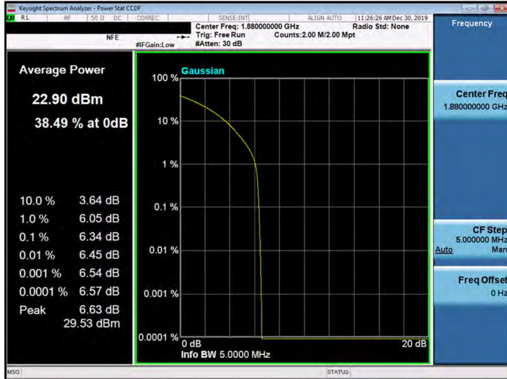
Plot 7-435. PAR Plot (5G NR n2 - 5.0MHz QPSK - CP - CP - Full RB Configuration)
