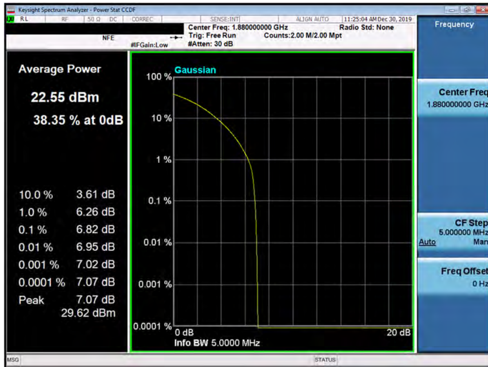
Plot 7-437. PAR Plot (5G NR n2 - 5.0MHz 64-QAM - CP - Full RB Configuration)
