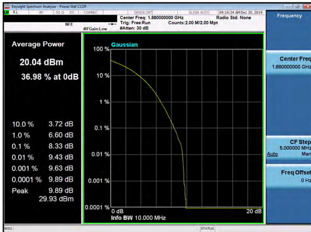
Plot 7-442. PAR Plot (5G NR n2 - 10.0MHz 256-QAM - CP - Full RB Configuration)
