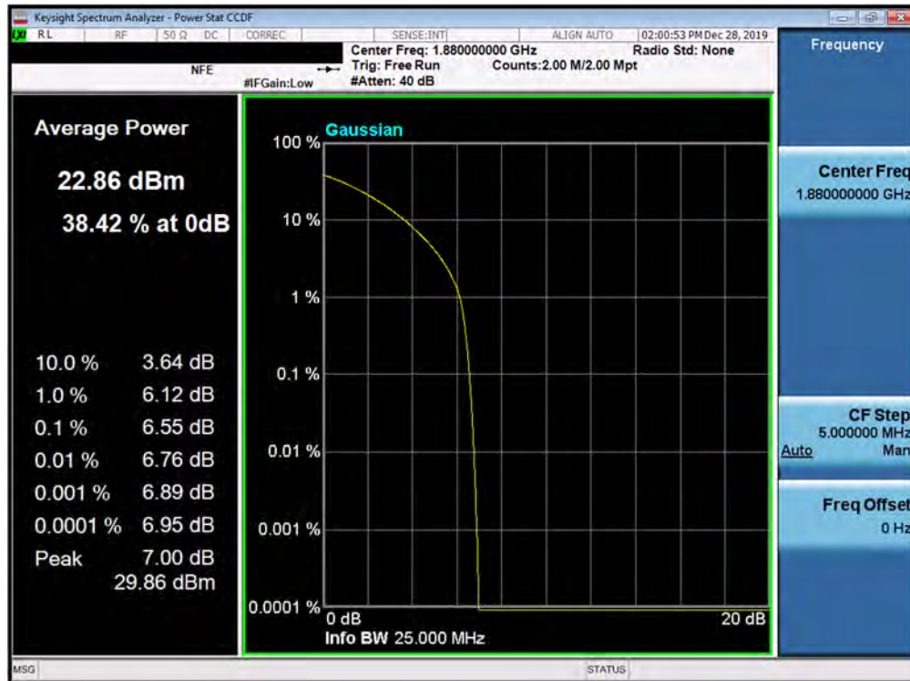
Plot 7-443. PAR Plot (5G NR n2 - 15.0MHz QPSK - CP - CP - Full RB Configuration)
