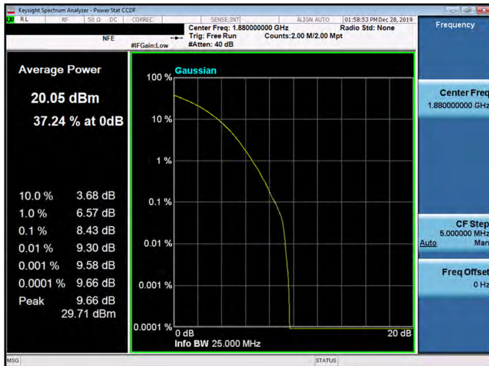
Plot 7-446. PAR Plot (5G NR n2 - 15.0MHz 256-QAM - CP - Full RB Configuration)
