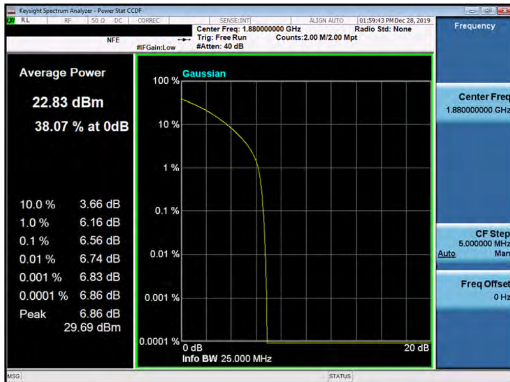
Plot 7-444. PAR Plot (5G NR n2 - 15.0MHz 16-QAM - CP - Full RB Configuration)
