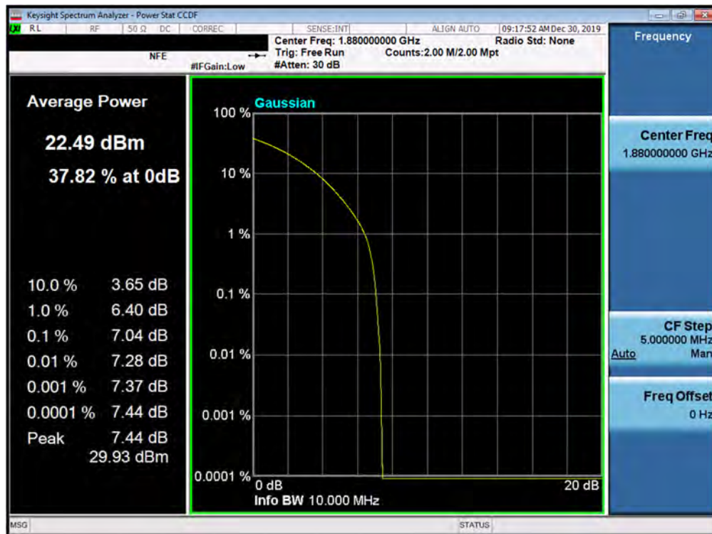
Plot 7-441. PAR Plot (5G NR n2 - 10.0MHz 64-QAM - CP - Full RB Configuration)
