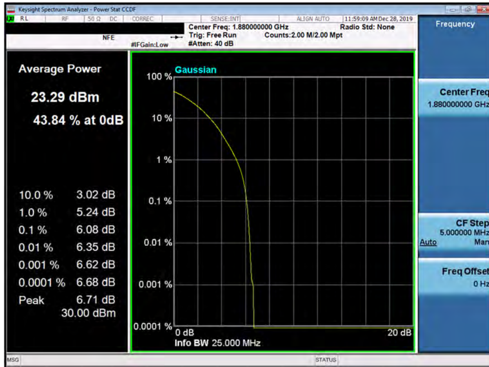
Plot 7-449. PAR Plot (5G NR n2 - 20.0MHz 64-QAM - CP - Full RB Configuration)
