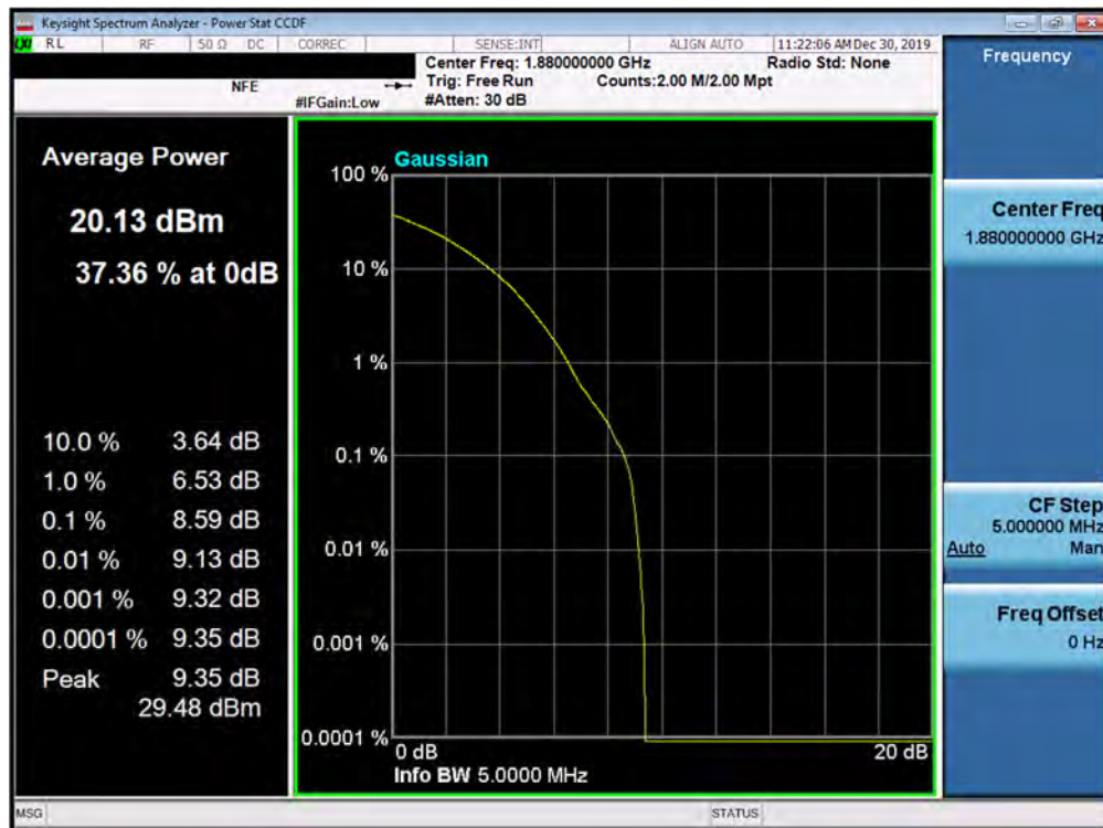
Plot 7-438. PAR Plot (5G NR n2 - 5.0MHz 256-QAM - CP - Full RB Configuration)
