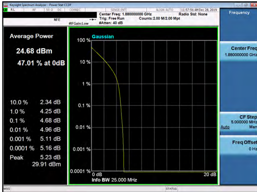
Plot 7-447. PAR Plot (5G NR n2 - 20.0MHz QPSK - CP - CP - Full RB Configuration)
