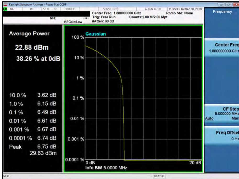
Plot 7-436. PAR Plot (5G NR n2 - 5.0MHz 16-QAM - CP - Full RB Configuration)
