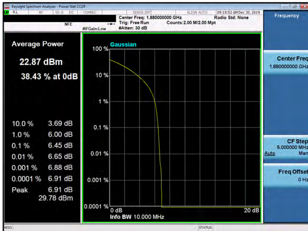
Plot 7-440. PAR Plot (5G NR n2 - 10.0MHz 16-QAM - CP - Full RB Configuration)
