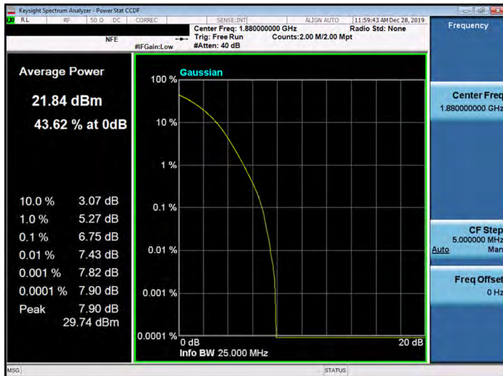
Plot 7-450. PAR Plot (5G NR n2 - 20.0MHz 256-QAM - CP - Full RB Configuration)
