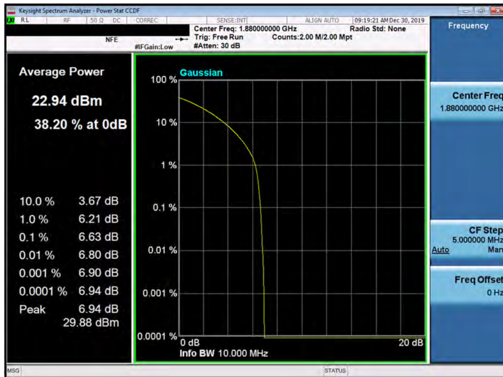
Plot 7-439. PAR Plot (5G NR n2 - 10.0MHz QPSK - CP - CP - Full RB Configuration)
