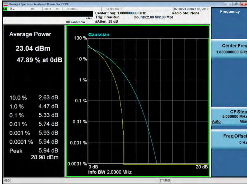
Plot 7-411. PAR Plot (Band 2 - 1.4MHz QPSK - Full RB Configuration)
