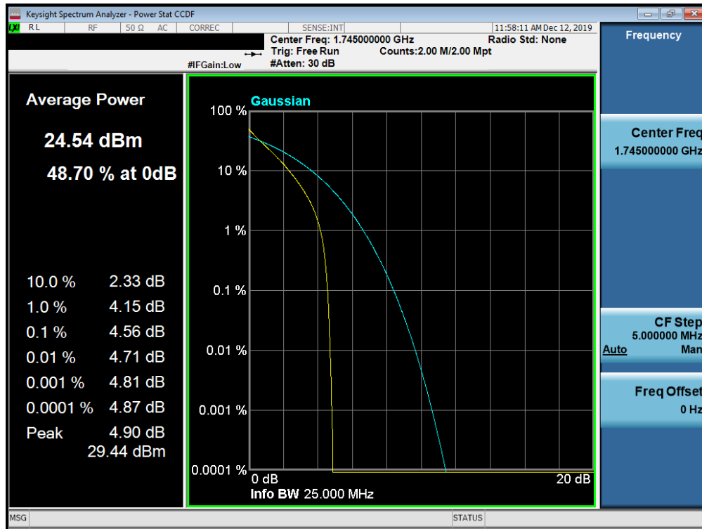
Plot 7-765. PAR Plot (Band n66 - 20.0MHz QPSK - Full RB Configuration)
