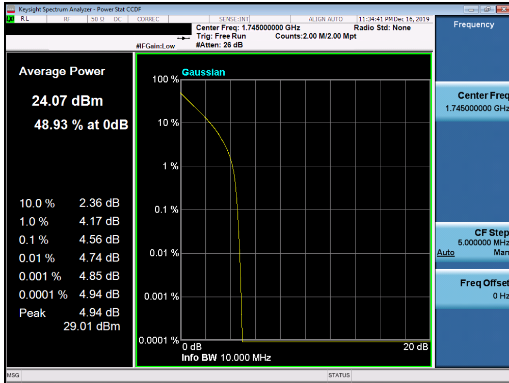
Plot 7-757. PAR Plot (Band n66 - 10.0MHz QPSK - Full RB Configuration)
