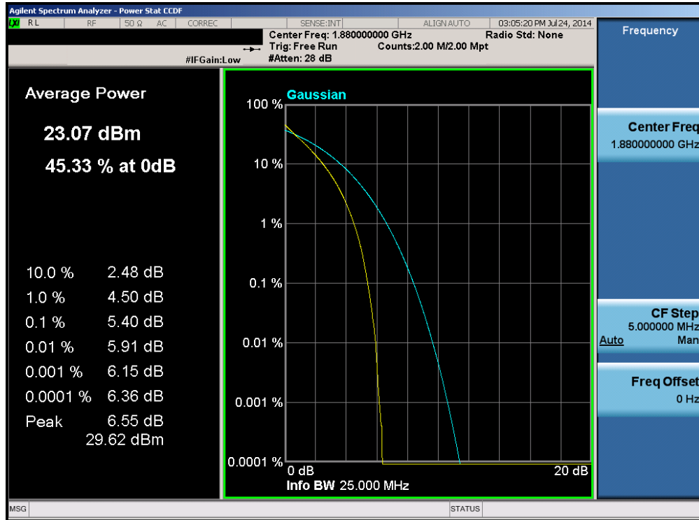
Plot 6-101. PAR Plot (Band 2 – 20.0MHz QPSK – RB Size 100)
