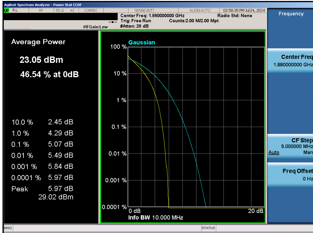
Plot 6-97. PAR Plot (Band 2 – 10.0MHz QPSK – RB Size 50)
