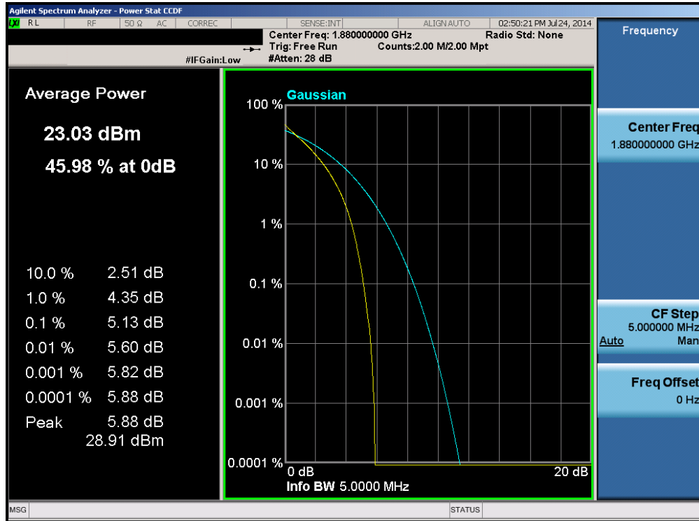
Plot 6-95. PAR Plot (Band 2 – 5.0MHz QPSK – RB Size 25)
