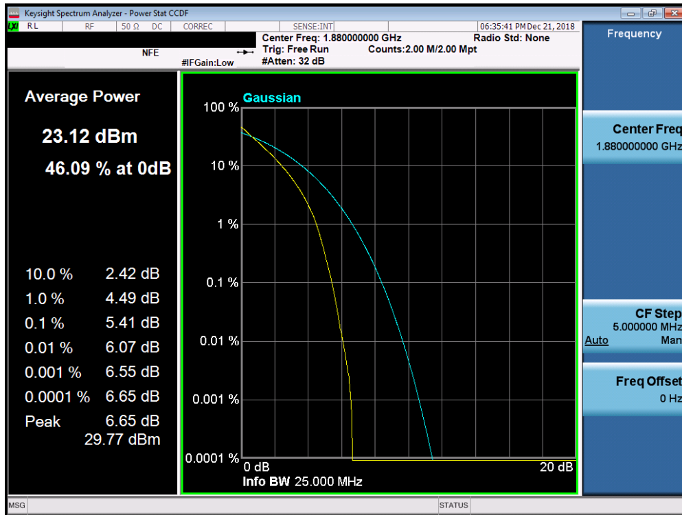
Plot 7-259. PAR Plot (Band 2/25 - 15.0MHz QPSK - Full RB Configuration)
