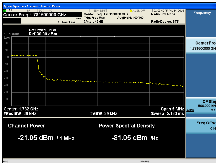
LTE Band 4,66 / 5MHz / QPSK - RB Size/Offset (25/0)
