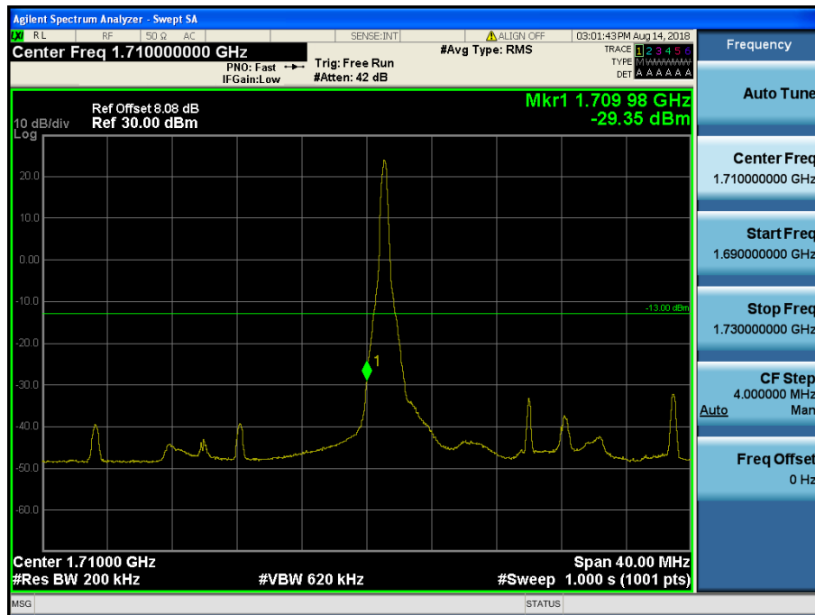
LTE Band 4,66 / 20MHz / QPSK - RB Size/Offset (1/0)
