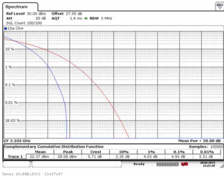
PAR Plot (21100 ch_5 MHz_QPSK_RB 25)
