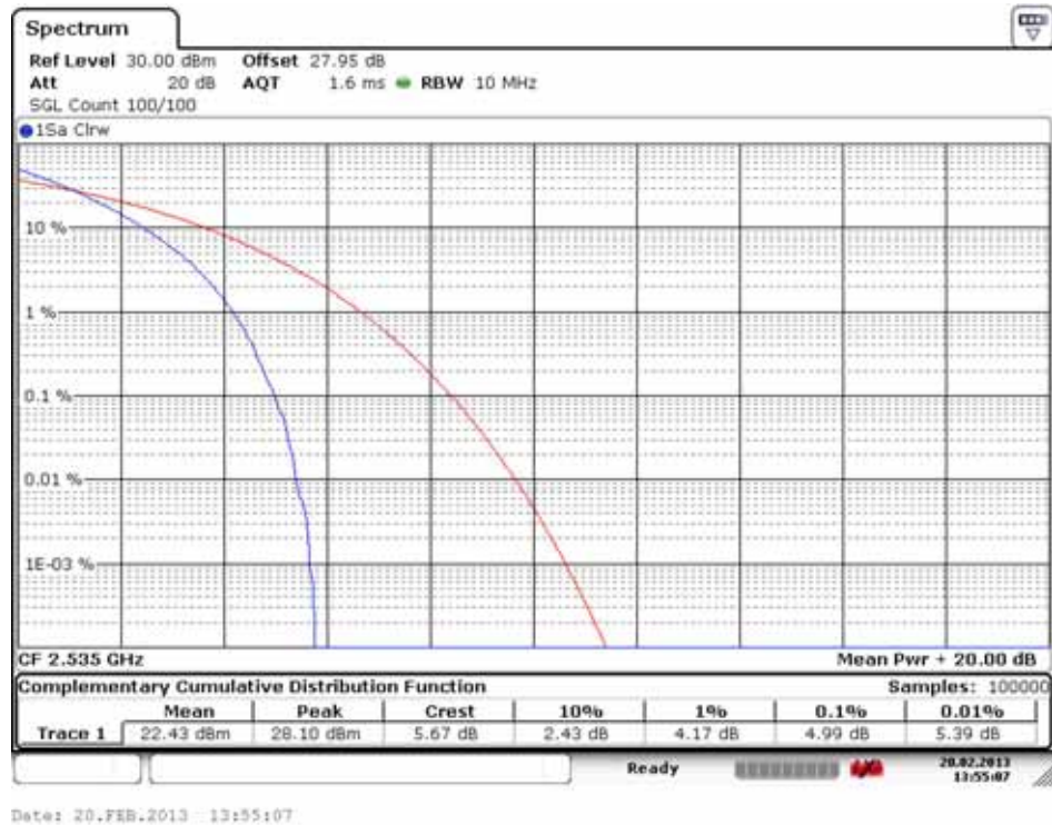
PAR Plot (21100 ch_10 MHz_QPSK_RB 50)
