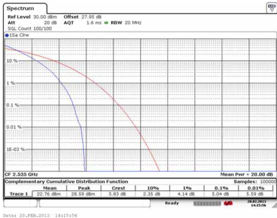
PAR Plot (21100 ch_15 MHz_QPSK_RB 75)
