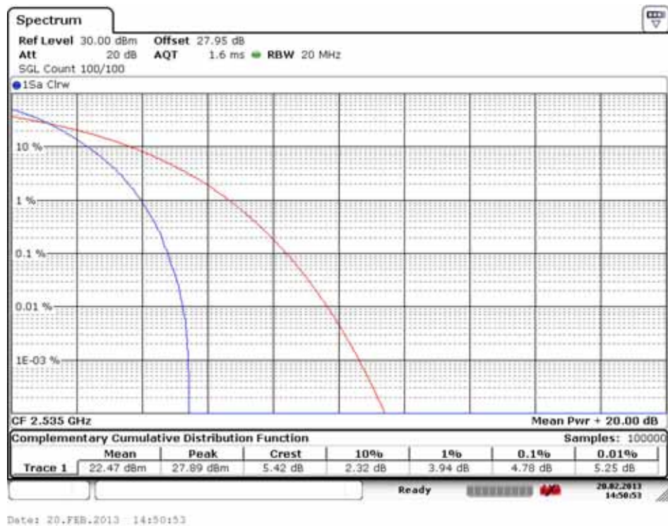
PAR Plot (21100 ch_20 MHz_QPSK_RB 100)
