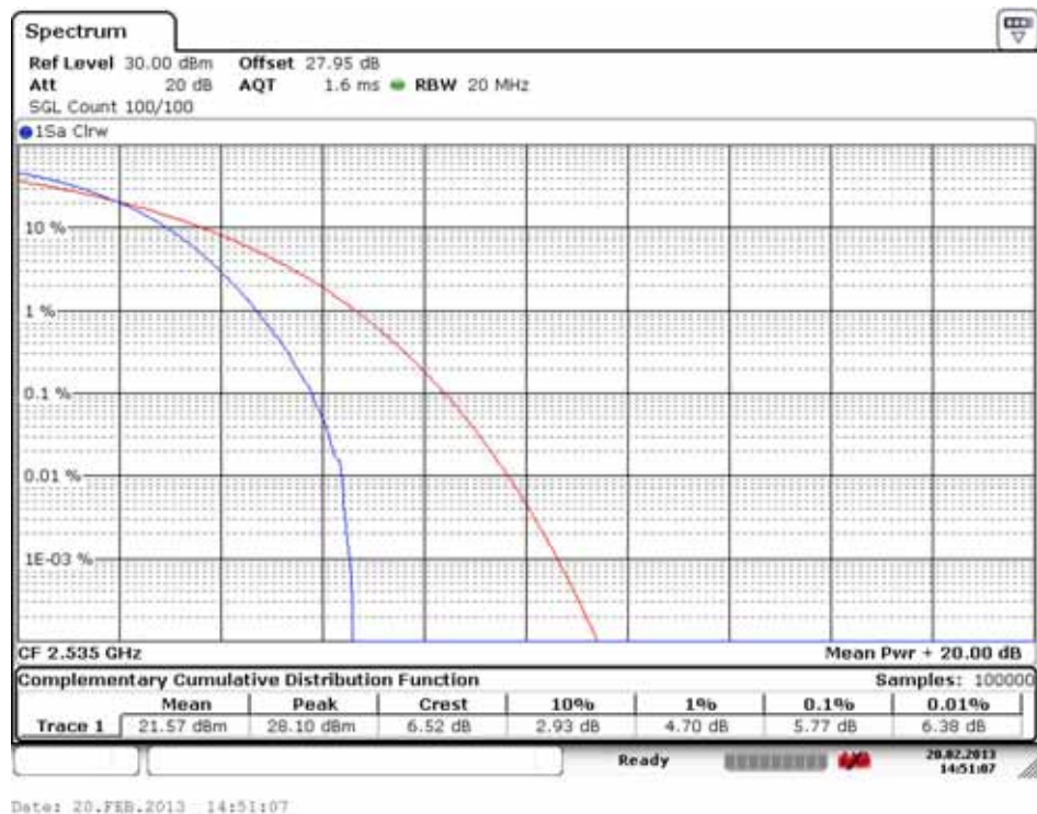
PAR Plot (21100 ch_20 MHz_16-QAM_RB 100)
