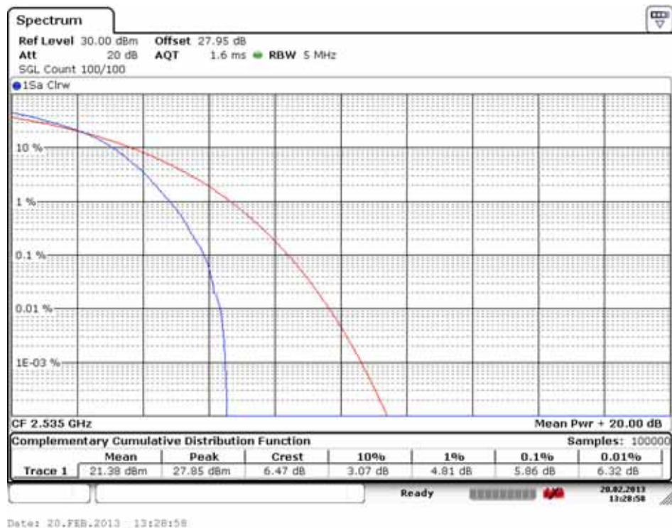
PAR Plot (21100 ch_5 MHz_16-QAM_RB 25)
