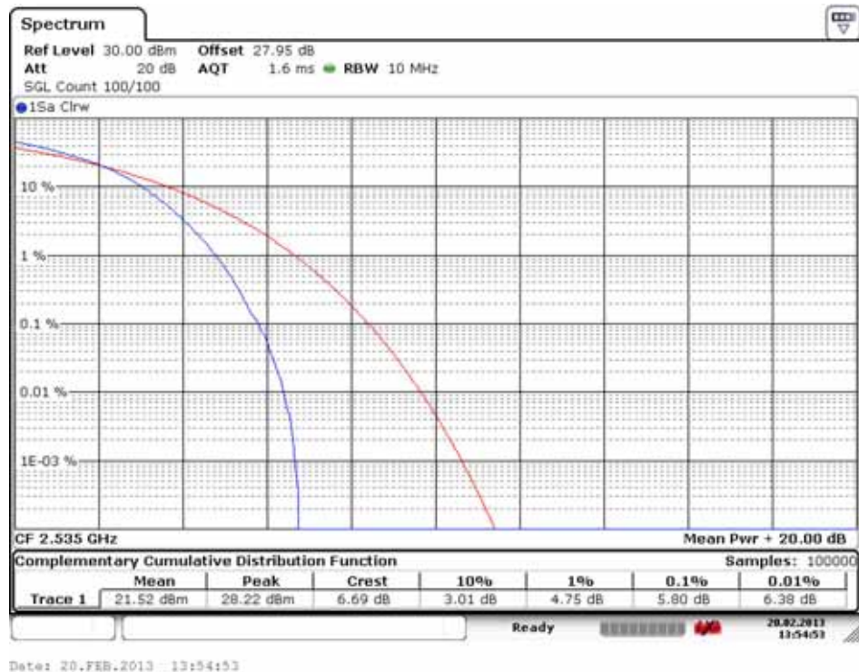
PAR Plot (21100 ch_10 MHz_16-QAM_RB 50)
