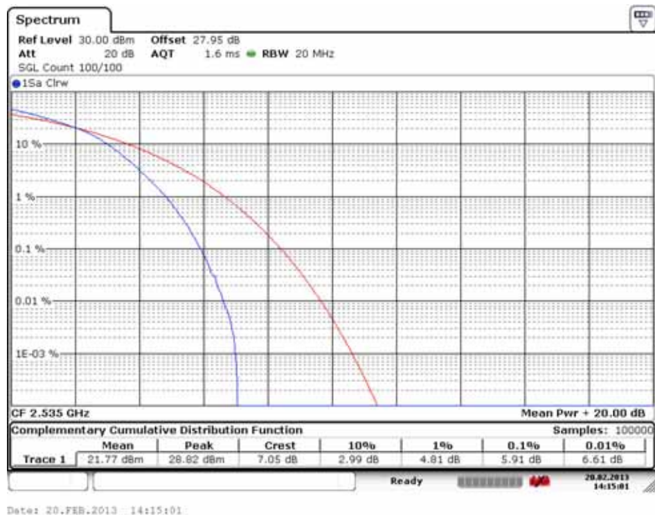
PAR Plot (21100 ch_15 MHz_16-QAM_RB 75)
