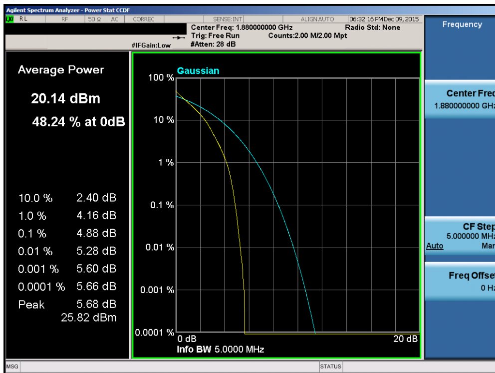
Plot 7-117. PAR Plot (Band 2 – 5.0MHz QPSK – RB Size 25)
