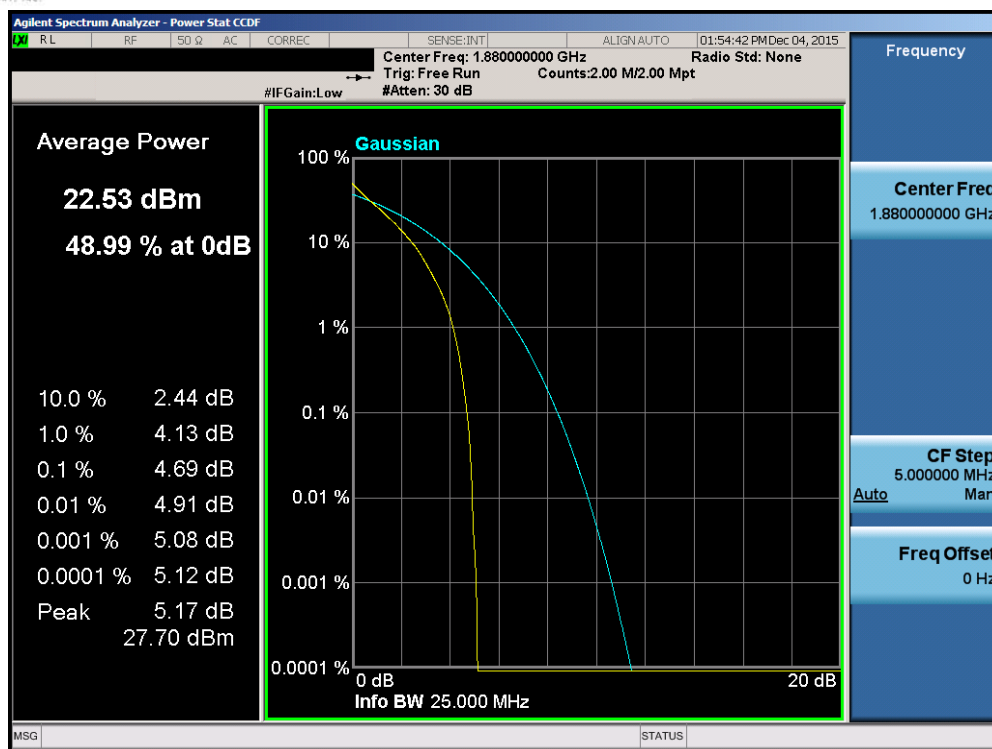
Plot 7-121. PAR Plot (Band 2 – 15.0MHz QPSK – RB Size 75)
