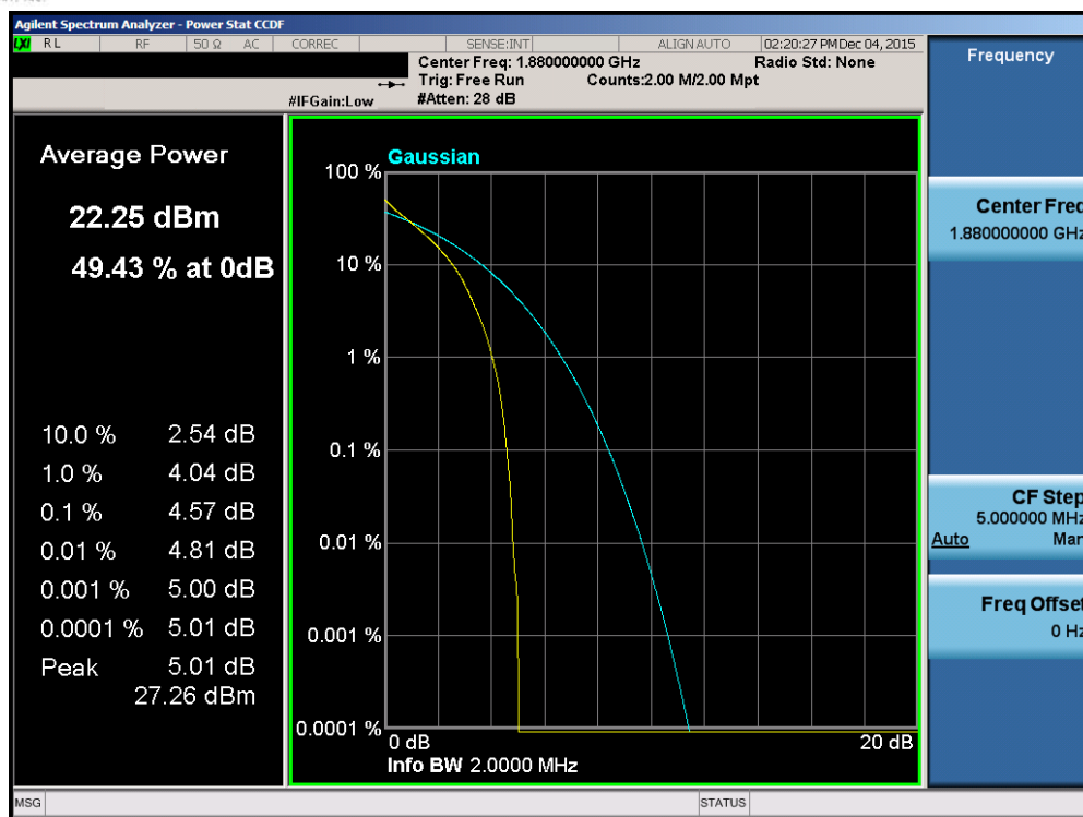
Plot 7-113. PAR Plot (Band 2 – 1.4MHz QPSK – RB Size 6)
