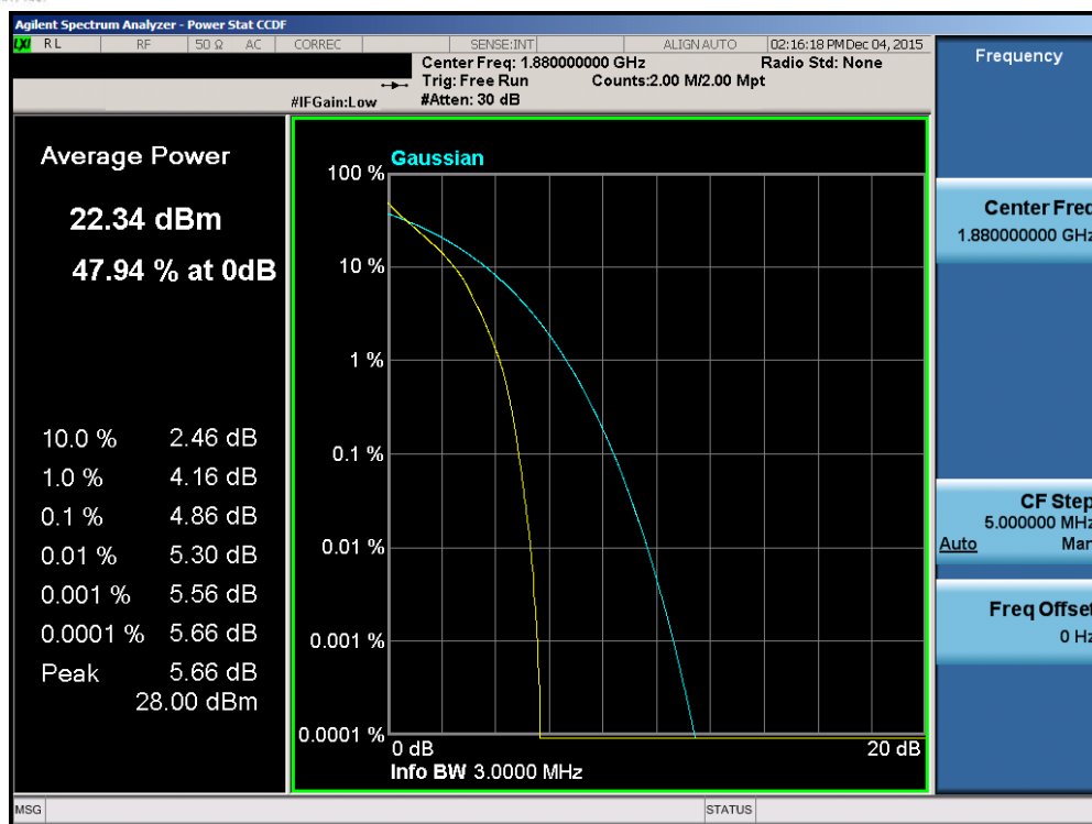
Plot 7-115. PAR Plot (Band 2 – 3.0MHz QPSK – RB Size 15)
