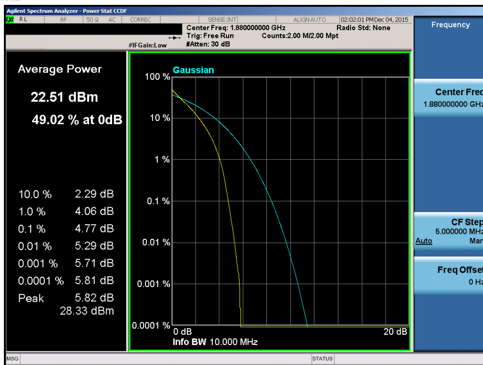
Plot 7-119. PAR Plot (Band 2 – 10.0MHz QPSK – RB Size 50)
