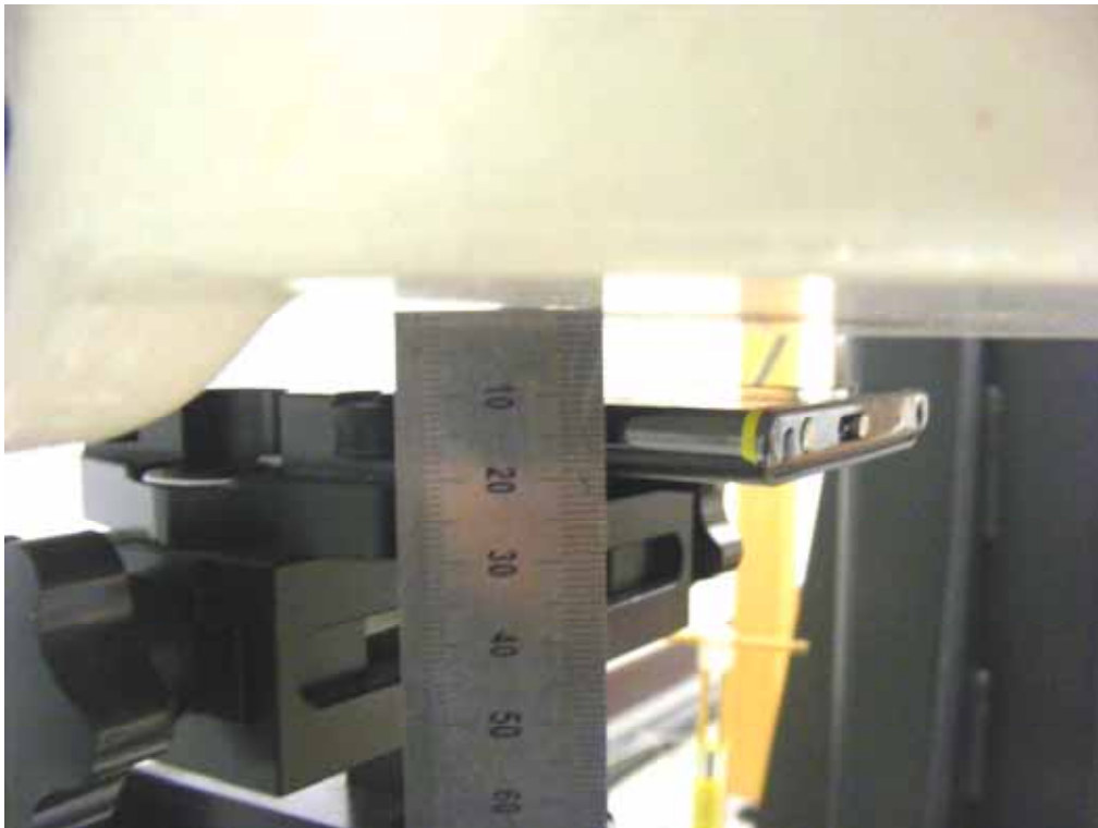
Body_Front (1 cm)
