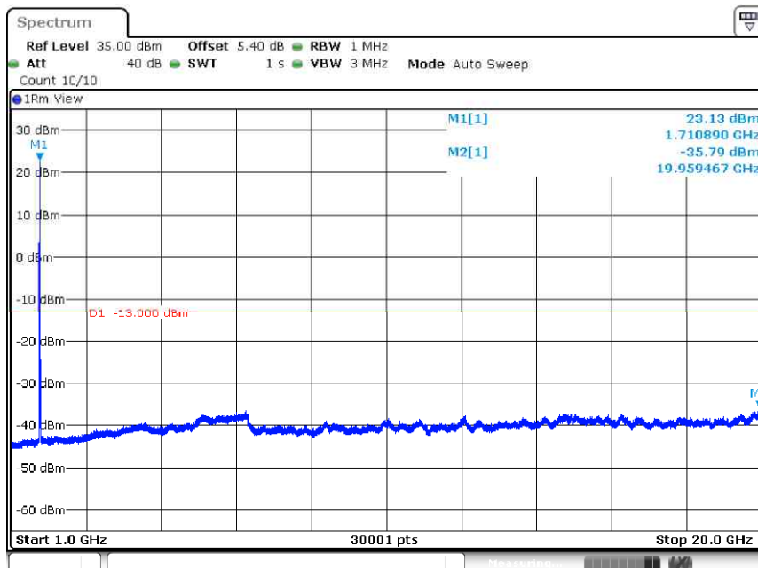
Band4-20MHz-QPSK-20050-1RB#0-Range2:1000~20000MHz
