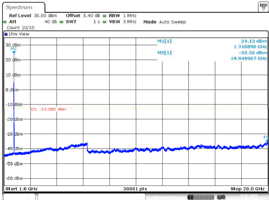
Band66-20MHz-QPSK-132072-1RB#0-Range2:1000~20000MHz
