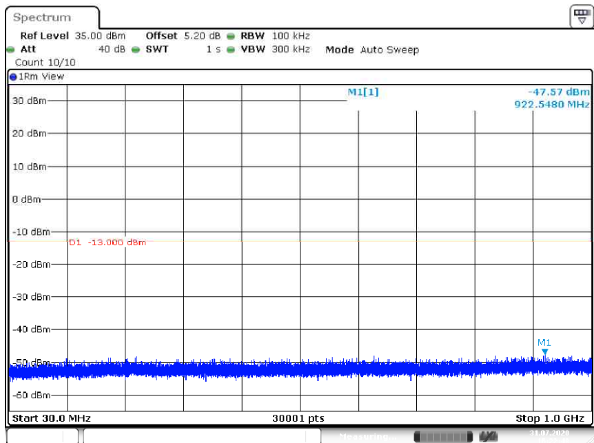
Band66-20MHz-QPSK-132072-1RB#0-Range1:30~1000MHz
