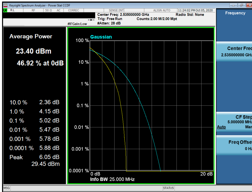
Plot 7-30. PAR Plot (LTE Band 7 - 20MHz QPSK - Full RB Configuration)
