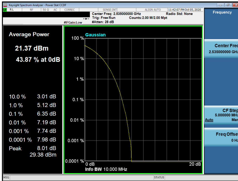
Plot 7 29. PAR Plot (LTE Band 7 - 10MHz 64-QAM - Full RB Configuration)
