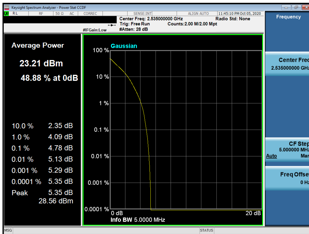
Plot 7-37. PAR Plot (LTE Band 7 - 5MHz QPSK - Full RB Configuration)
