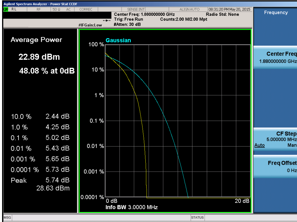
Plot 6-207. PAR Plot (Band 2 – 3.0MHz QPSK – RB Size 15)
