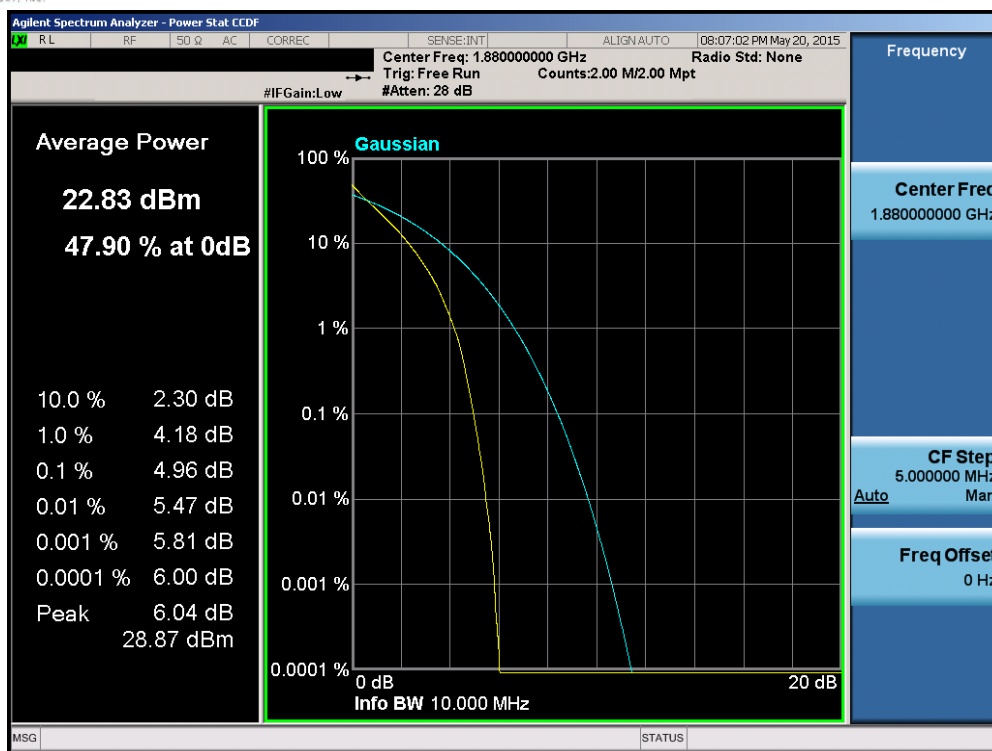
Plot 6-211. PAR Plot (Band 2 – 10.0MHz QPSK – RB Size 50)
