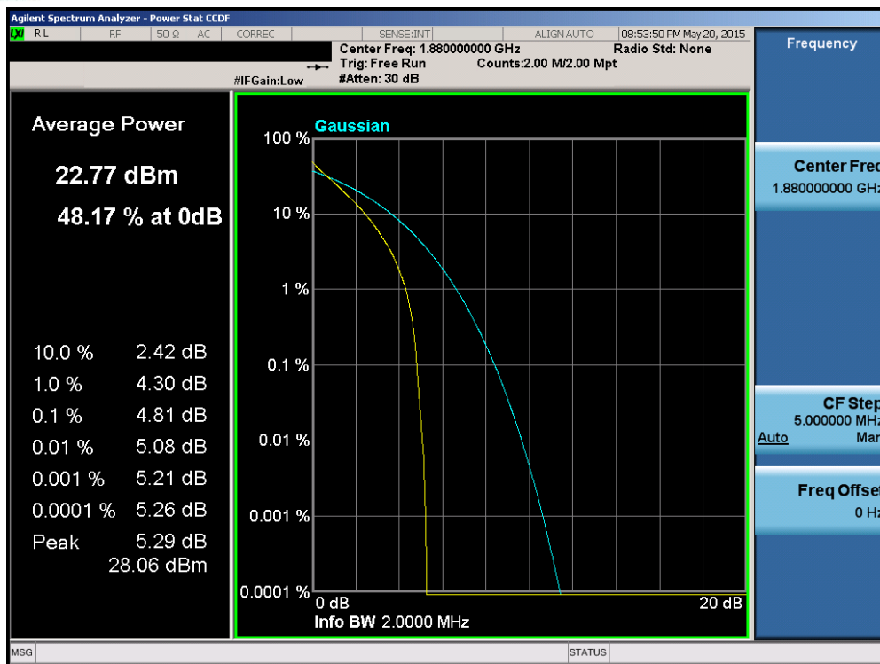
Plot 6-205. PAR Plot (Band 2 – 1.4MHz QPSK – RB Size 6)
