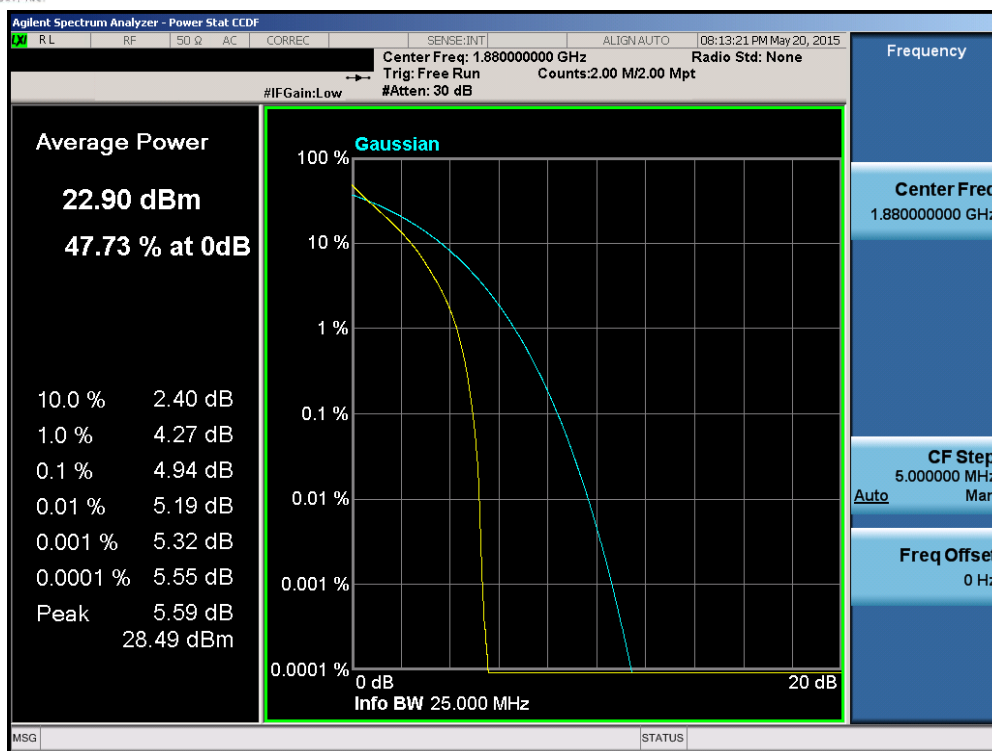
Plot 6-213. PAR Plot (Band 2 – 15.0MHz QPSK – RB Size 75)
