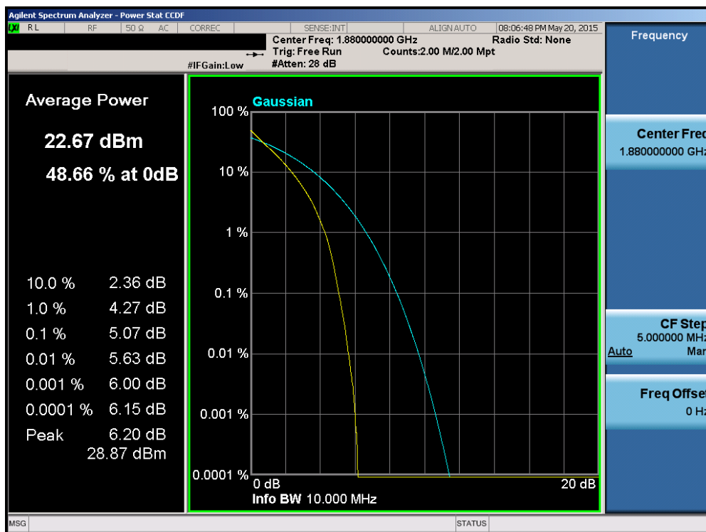
Plot 6-212. PAR Plot (Band 2 – 10.0MHz 16-QAM – RB Size 50)
