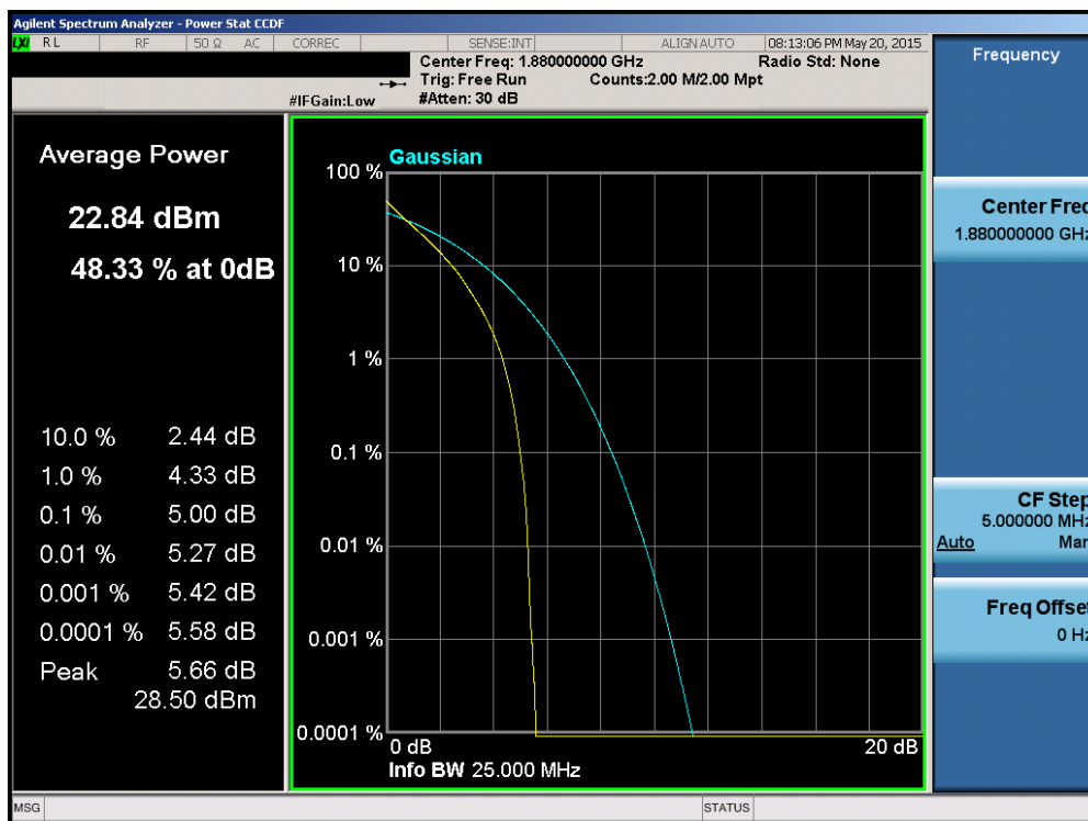
Plot 6-214. PAR Plot (Band 2 – 15.0MHz 16-QAM – RB Size 75)
