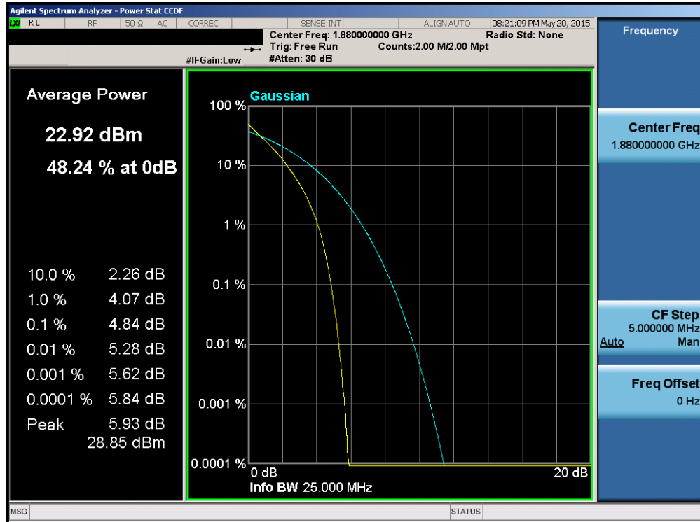
Plot 6-215. PAR Plot (Band 2 – 20.0MHz QPSK – RB Size 100)
