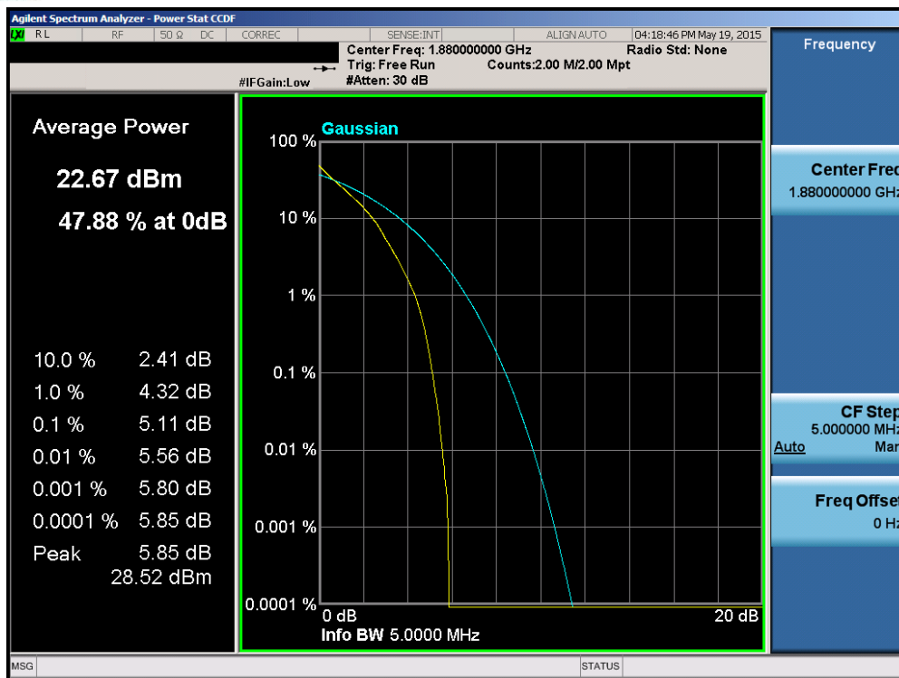
Plot 6-209. PAR Plot (Band 2 – 5.0MHz QPSK – RB Size 25)
