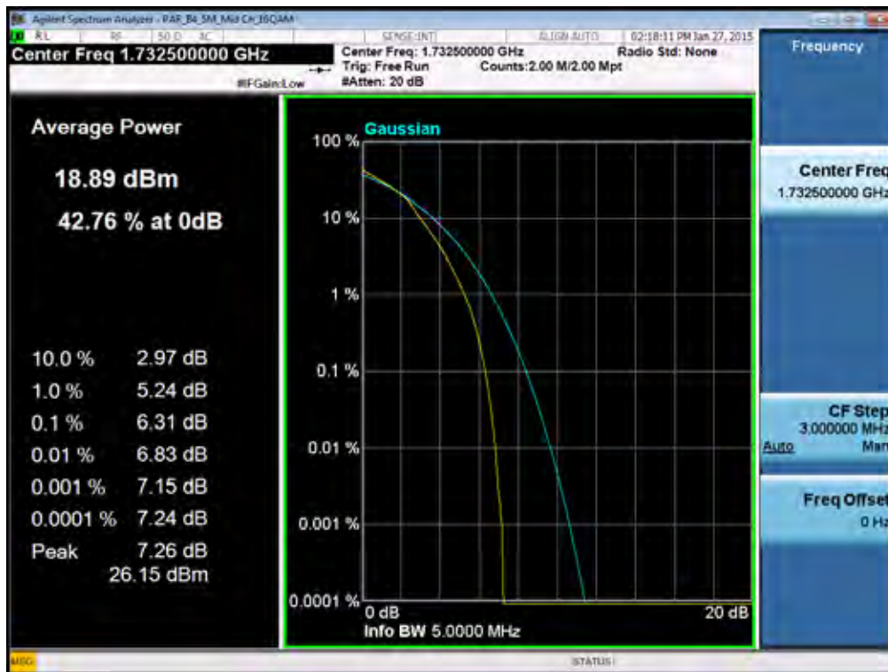
BAND 4. PAR Plot (5M BW_Ch.20175_16QAM_RB25_0)
