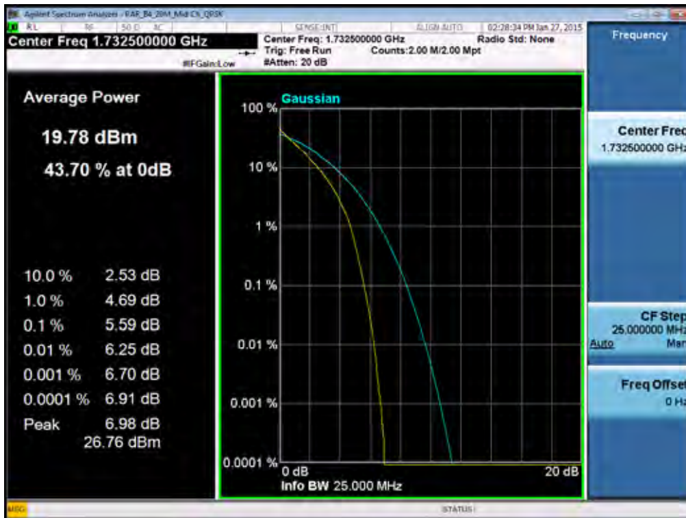
BAND 4. PAR Plot (20M BW_Ch.20175_QPSK_RB100_0)
