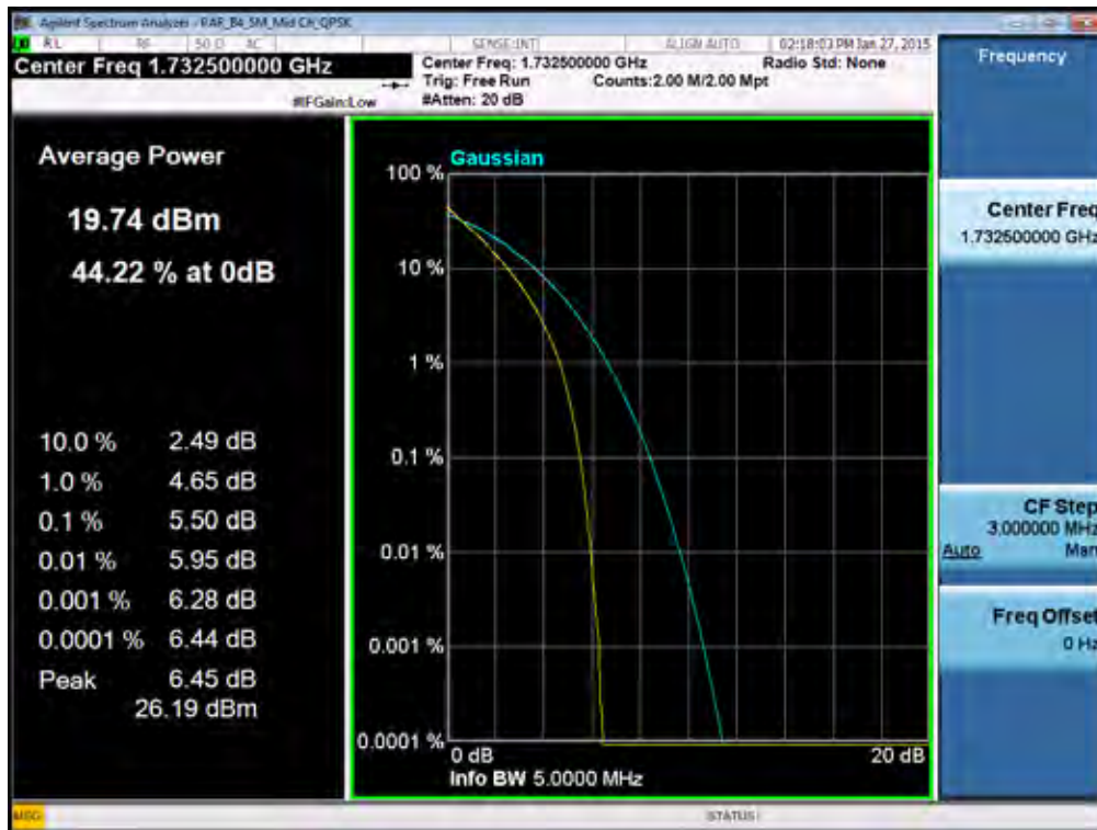
BAND 4. PAR Plot (5M BW_Ch.20175_QPSK_RB25_0)
