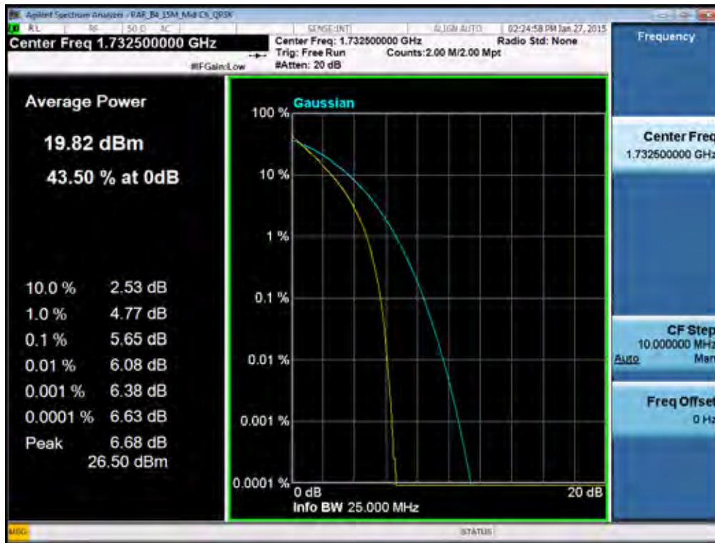
BAND 4. PAR Plot (15M BW_Ch.20175_QPSK_RB75_0)
