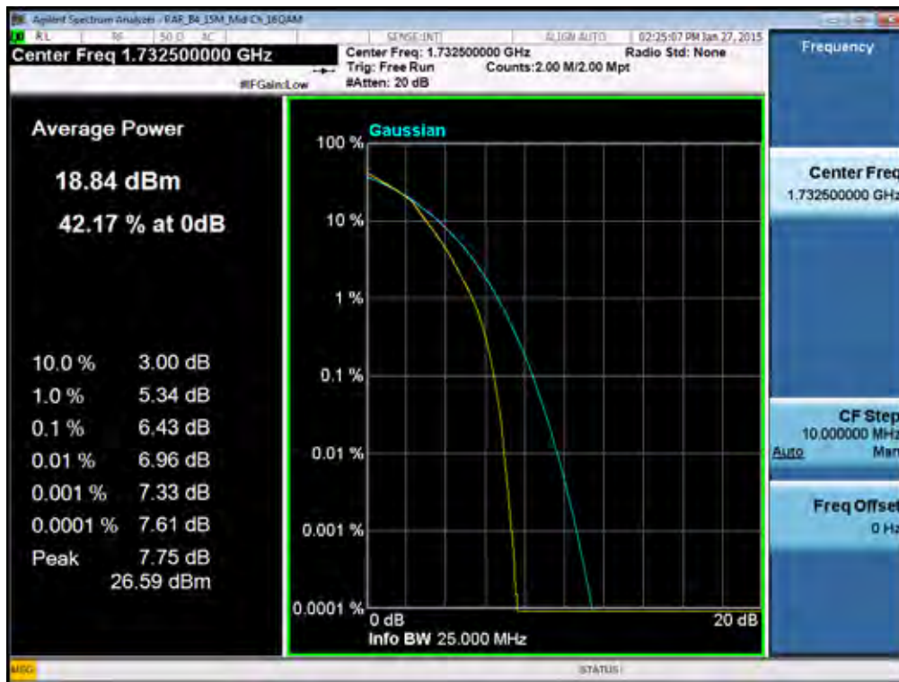
BAND 4. PAR Plot (15M BW_Ch.20175_16QAM_RB75_0)
