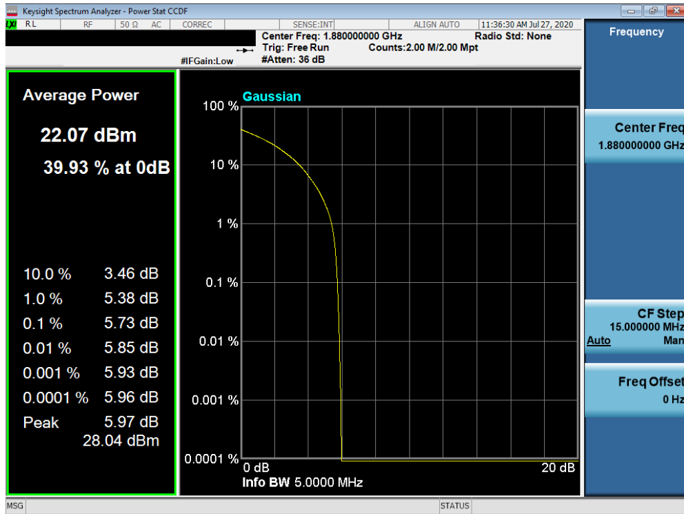
Plot 7-551. PAR Plot (NR n25/2 - 5.0MHz QPSK - Full RB Configuration)
