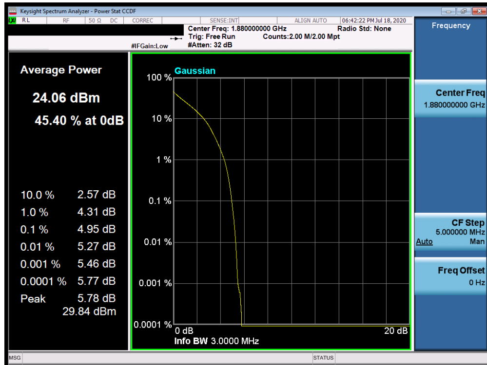
Plot 7-521. PAR Plot (Band 25/2 - 3.0MHz QPSK - Full RB Configuration)
