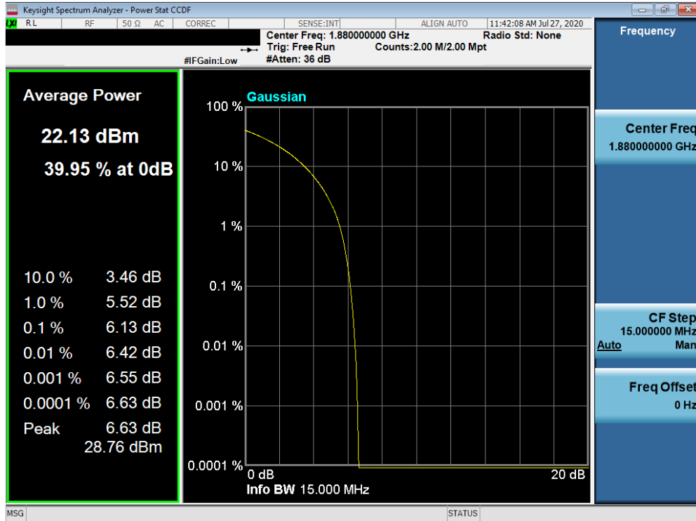
Plot 7-559. PAR Plot (NR n25/2 - 15.0MHz QPSK - Full RB Configuration)
