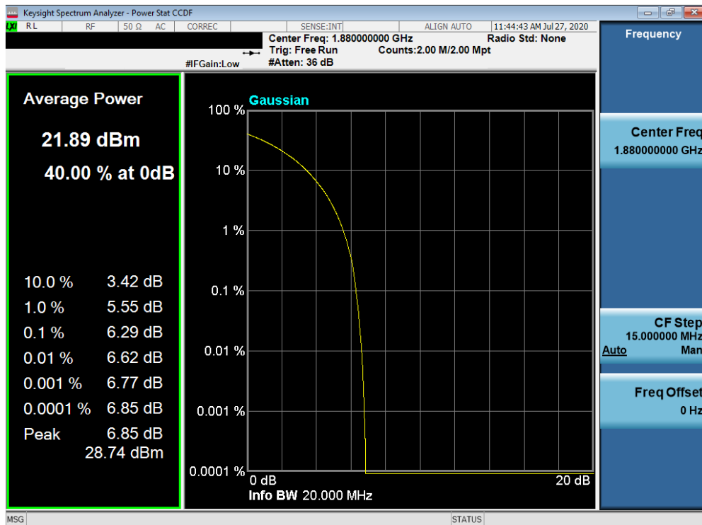
Plot 7-564. PAR Plot (NR n25/2 - 20.0MHz 16-QAM - Full RB Configuration)
