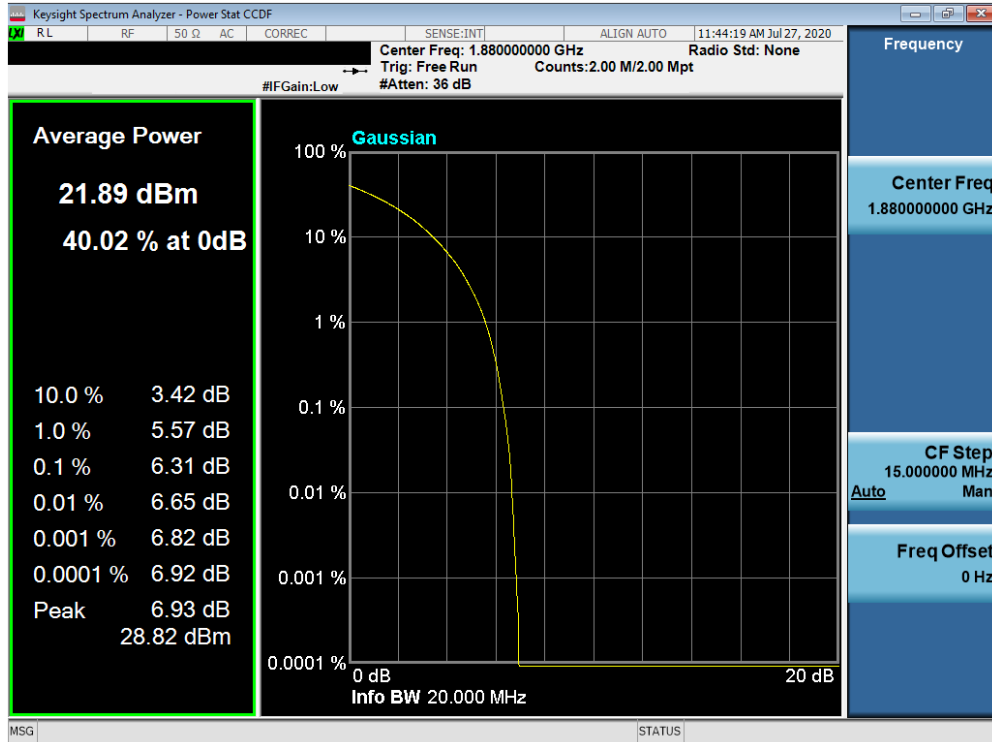
Plot 7-563. PAR Plot (NR n25/2 - 20.0MHz QPSK - Full RB Configuration)
