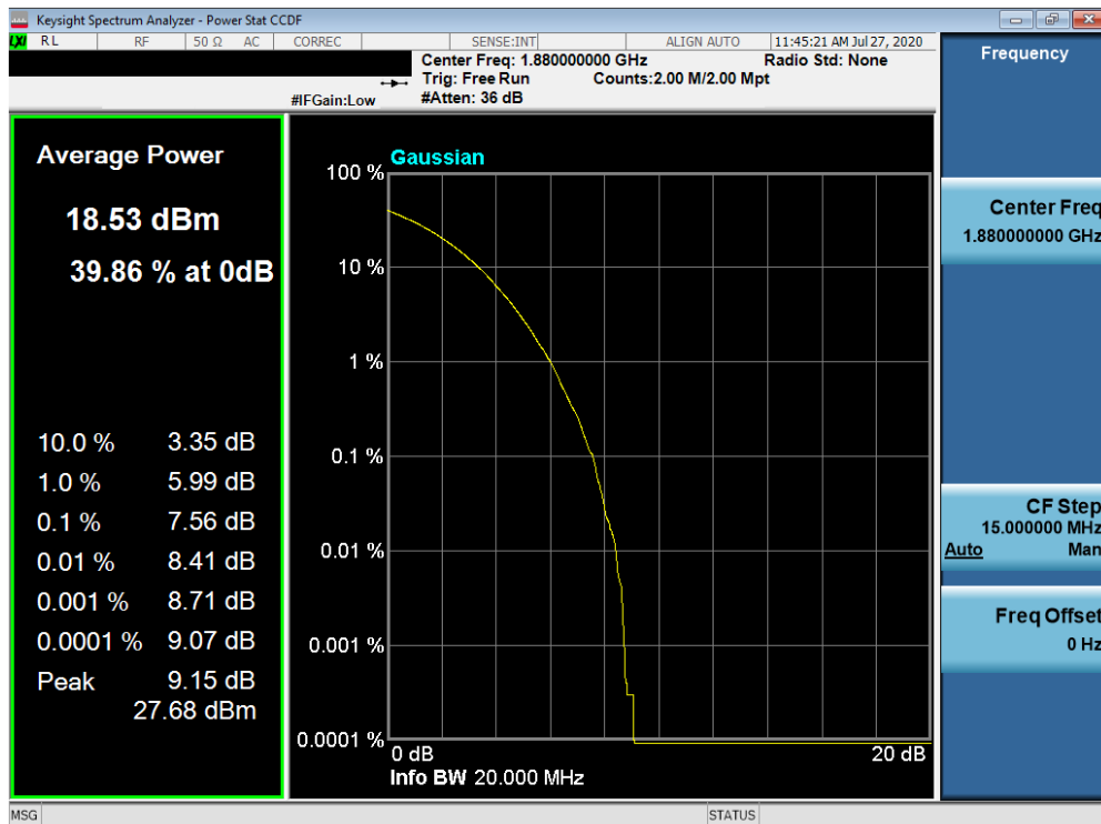
Plot 7-566. PAR Plot (NR n25/2 - 20.0MHz 256-QAM - Full RB Configuration)
