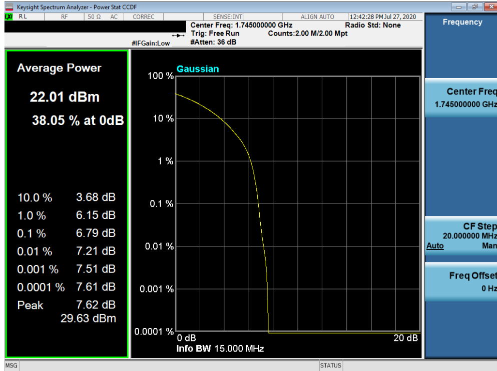
Plot 7-543. PAR Plot (NR n66/4 - 15.0MHz QPSK - Full RB Configuration)
