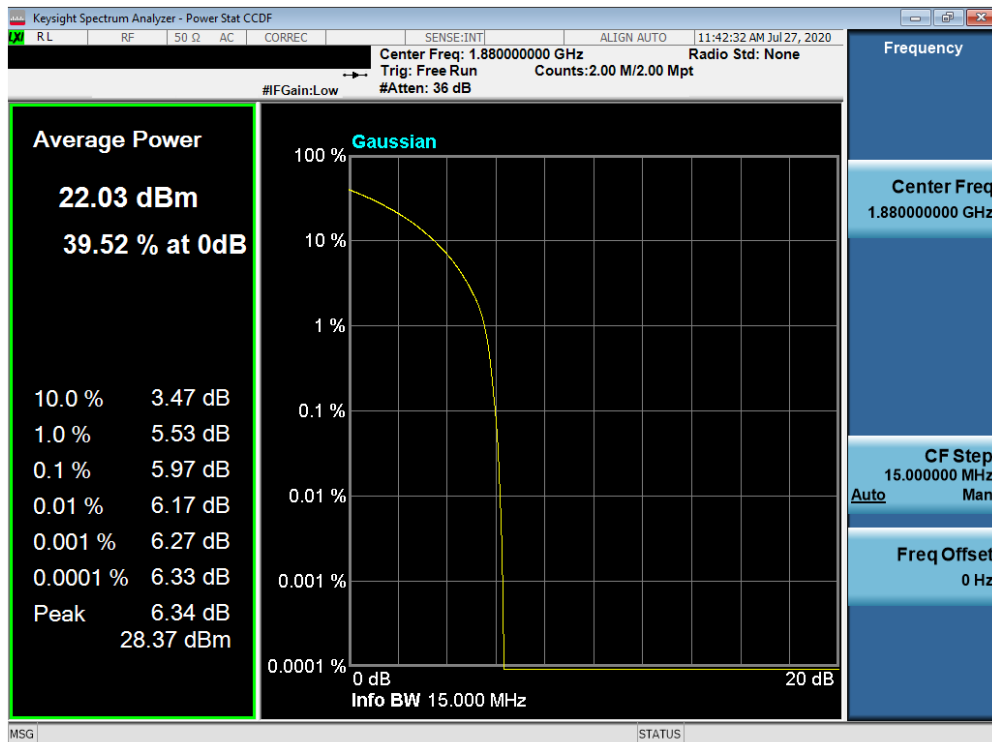
Plot 7-560. PAR Plot (NR n25/2 - 15.0MHz 16-QAM - Full RB Configuration)
