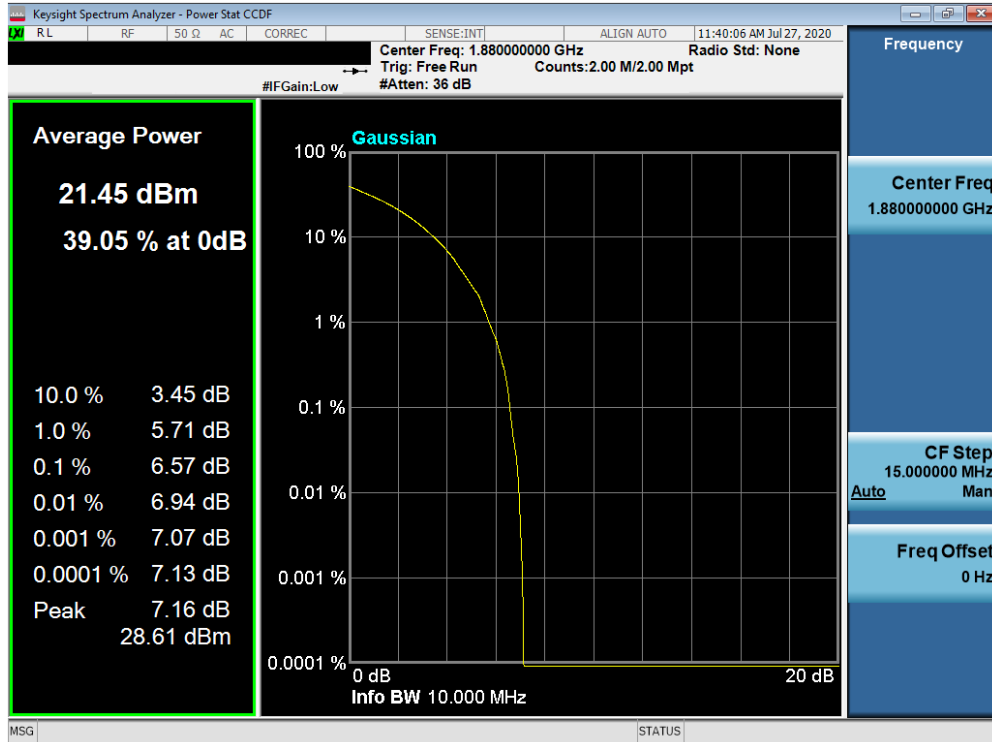
Plot 7-557. PAR Plot (NR n25/2 - 10.0MHz 64-QAM - Full RB Configuration)
