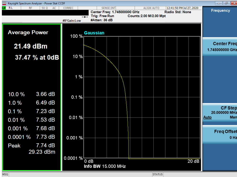
Plot 7-545. PAR Plot (NR n66/4 - 15.0MHz 64-QAM - Full RB Configuration)
