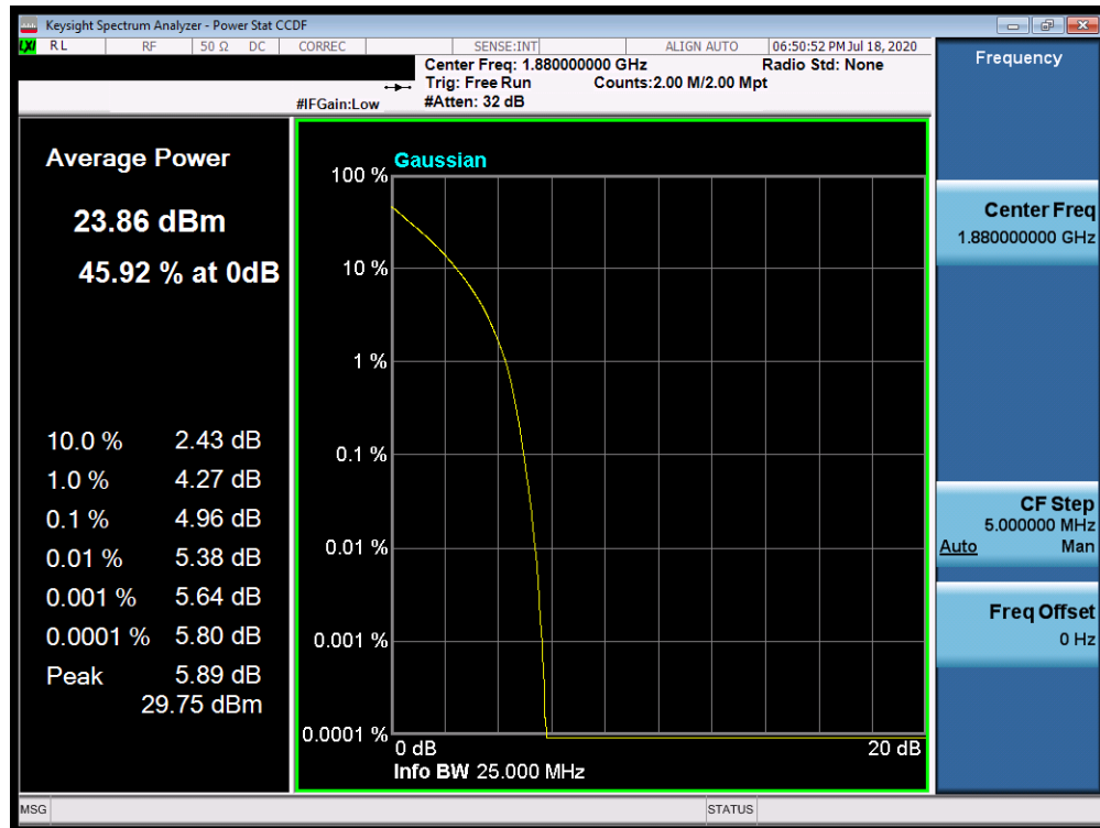
Plot 7-533. PAR Plot (Band 25/2 - 20.0MHz QPSK - Full RB Configuration)
