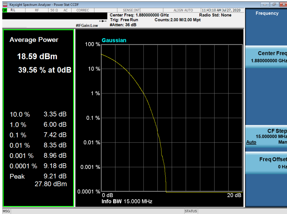
Plot 7-562. PAR Plot (NR n25/2 - 15.0MHz 256-QAM - Full RB Configuration)
