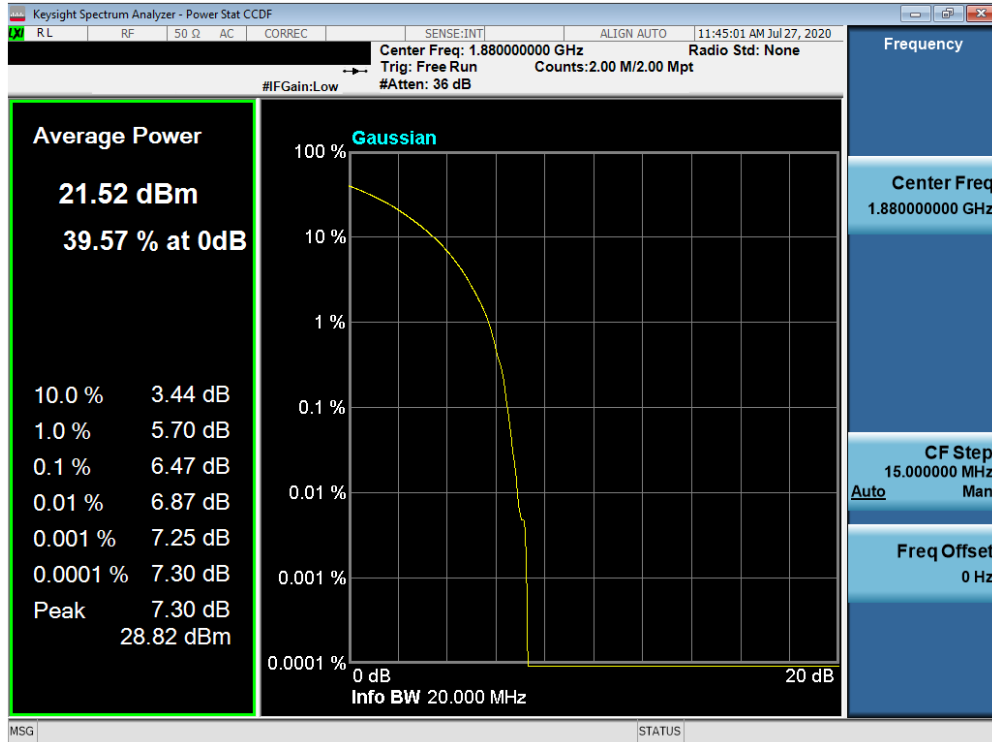
Plot 7-565. PAR Plot (NR n25/2 - 20.0MHz 64-QAM - Full RB Configuration)
