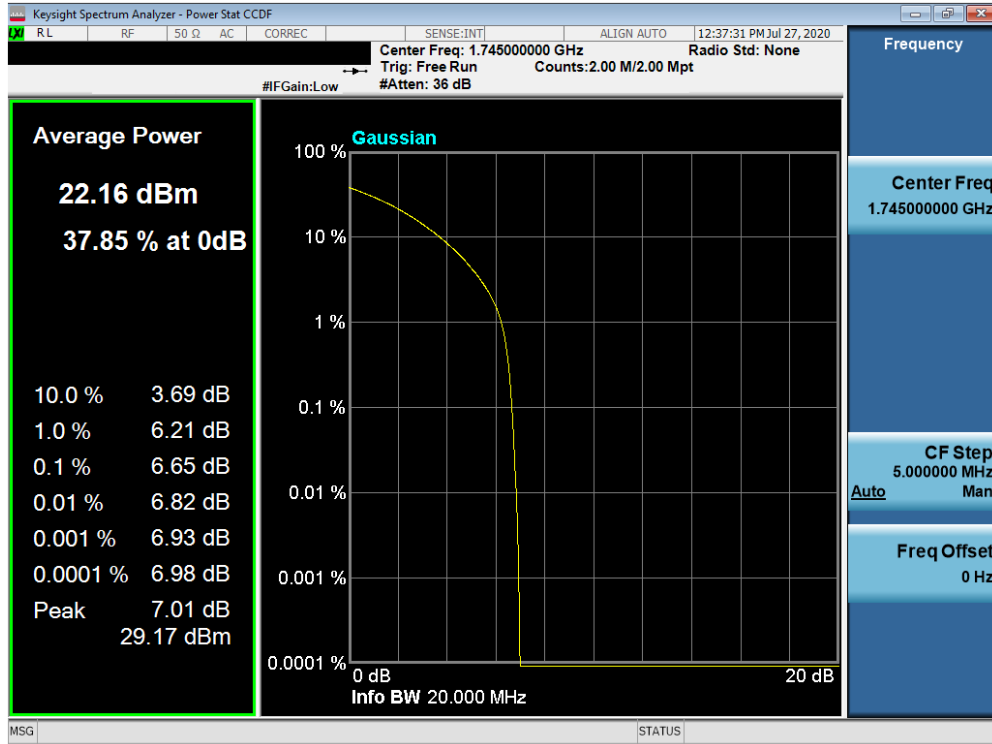
Plot 7-547. PAR Plot (NR n66/4 - 20.0MHz QPSK - Full RB Configuration)
