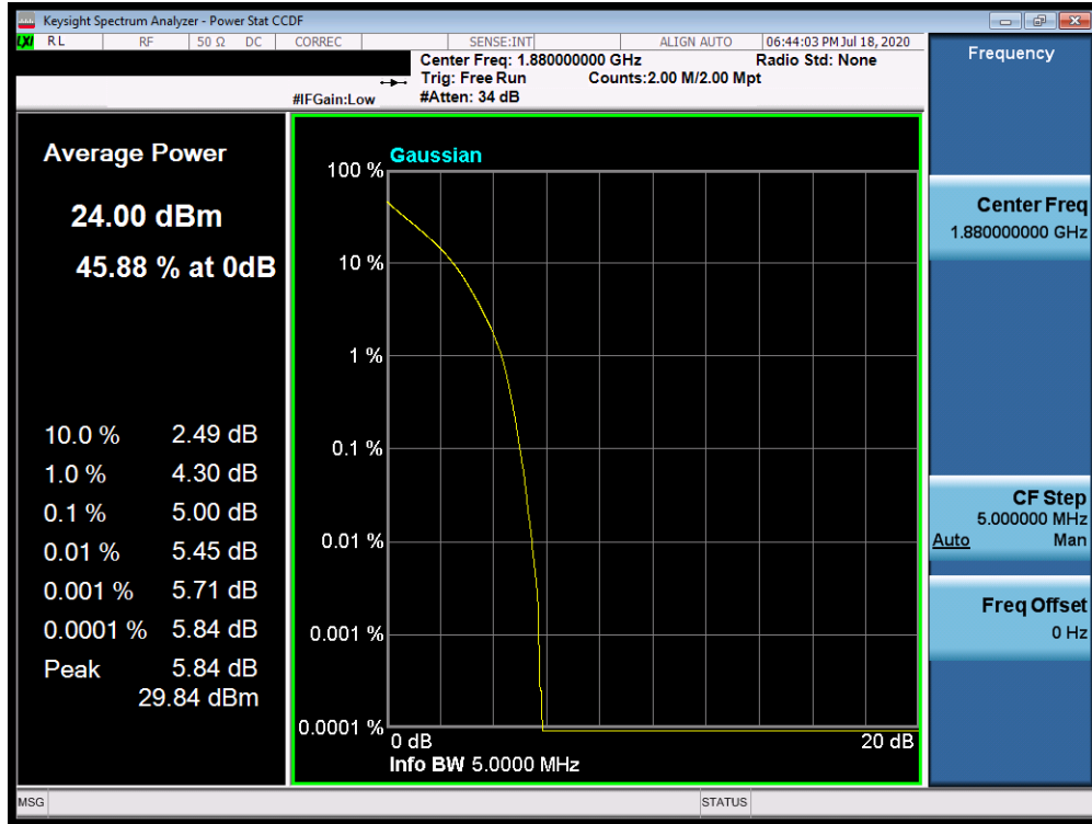
Plot 7-524. PAR Plot (Band 25/2 - 5.0MHz QPSK - Full RB Configuration)
