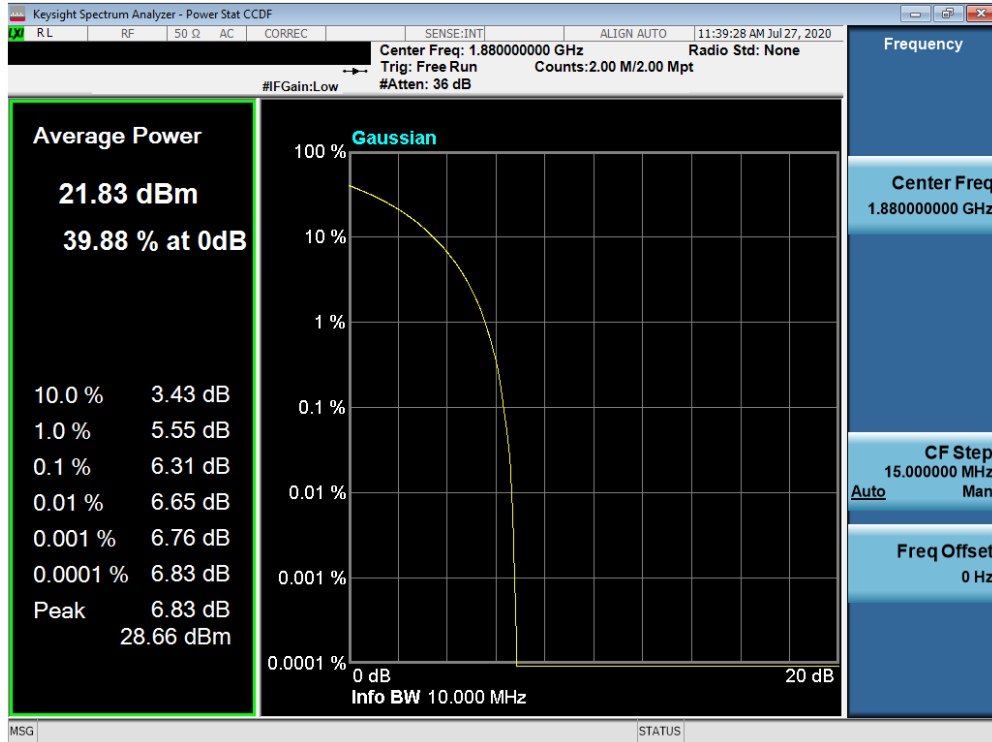
Plot 7-555. PAR Plot (NR n25/2 - 10.0MHz QPSK - Full RB Configuration)
