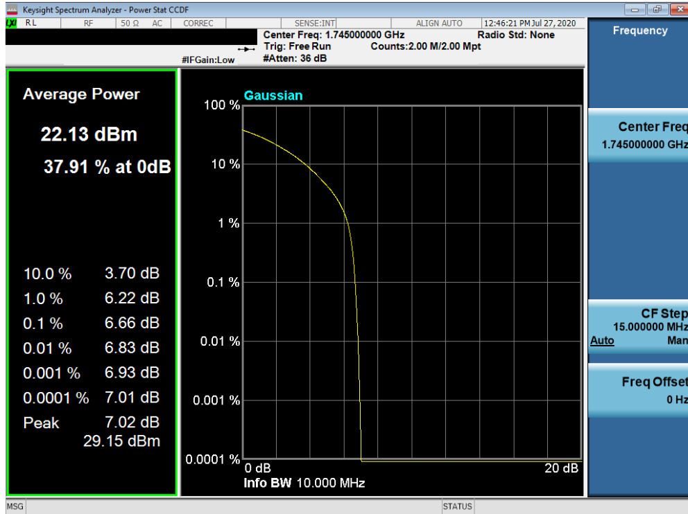
Plot 7-539. PAR Plot (NR n66/4 - 10.0MHz QPSK - Full RB Configuration)
