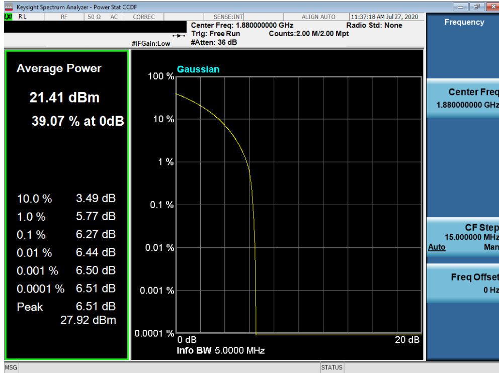
Plot 7-553. PAR Plot (NR n25/2 - 5.0MHz 64-QAM - Full RB Configuration)
