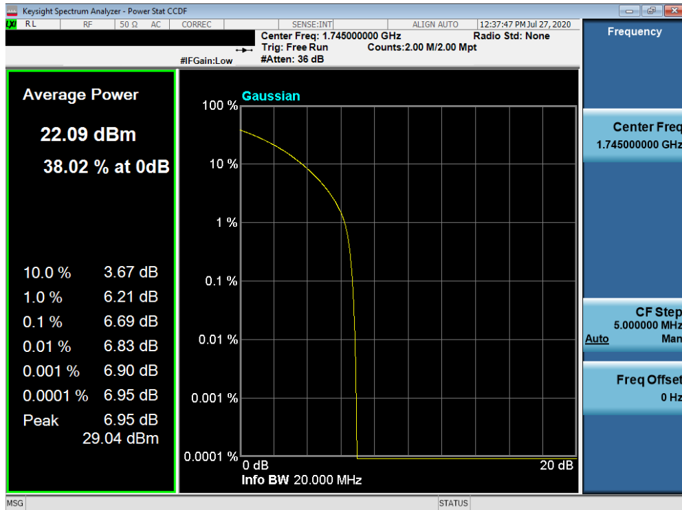
Plot 7-548. PAR Plot (NR n66/4 - 20.0MHz 16-QAM - Full RB Configuration)
