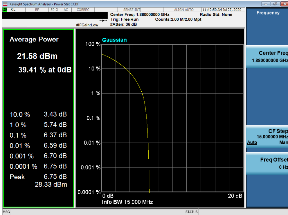
Plot 7-561. PAR Plot (NR n25/2 - 15.0MHz 64-QAM - Full RB Configuration)
