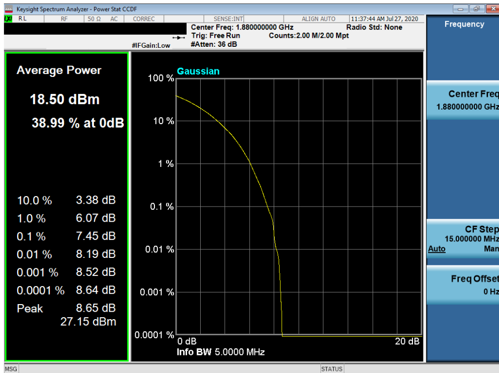
Plot 7-554. PAR Plot (NR n25/2 - 5.0MHz 256-QAM - Full RB Configuration)
