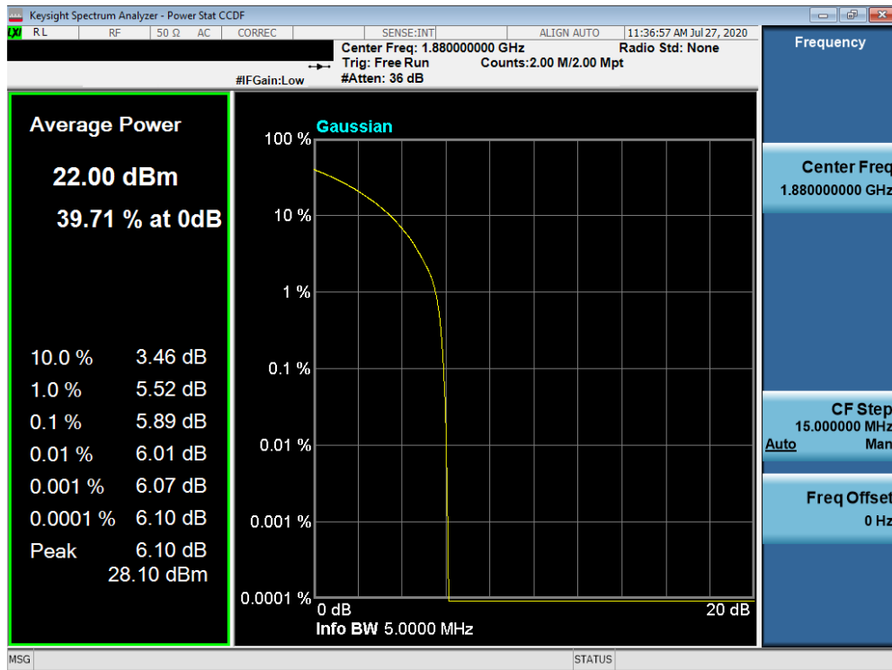
Plot 7-552. PAR Plot (NR n25/2 - 5.0MHz 16-QAM - Full RB Configuration)
