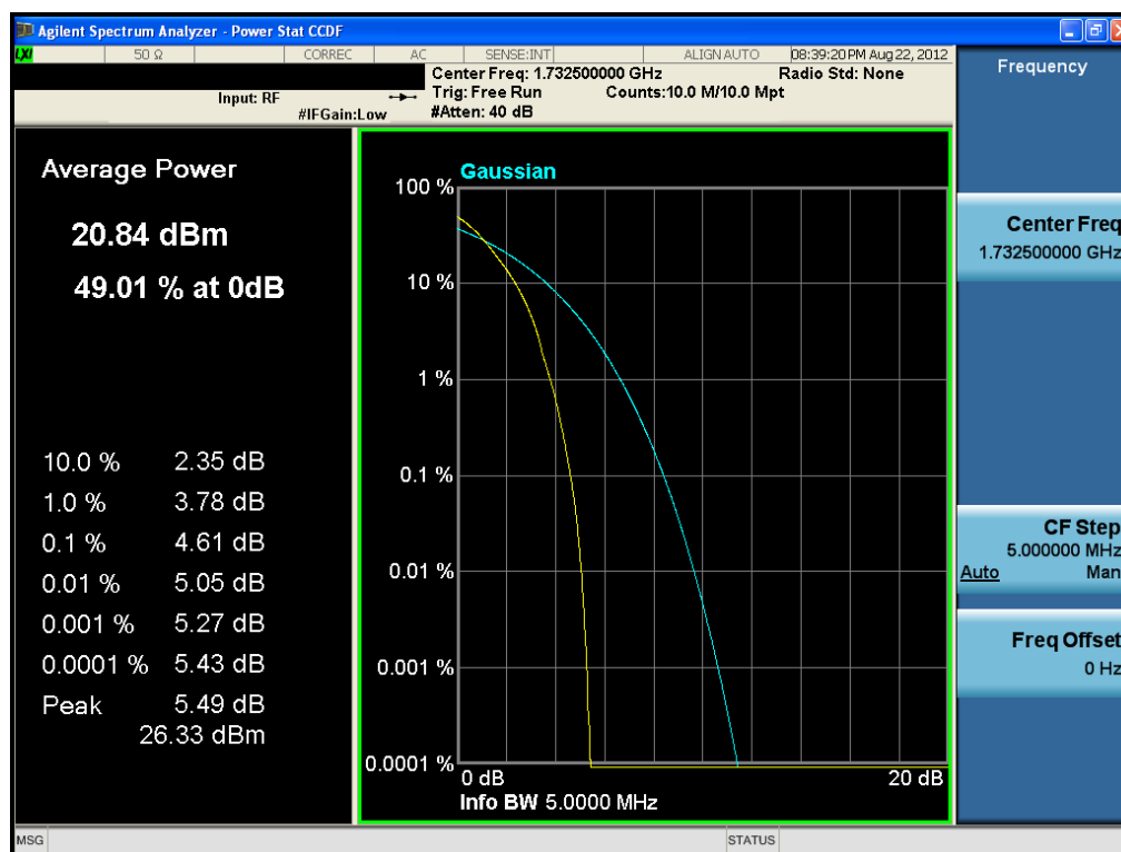
Plot 9-25. PAR Plot (5MHz QPSK – RB Size 25)
