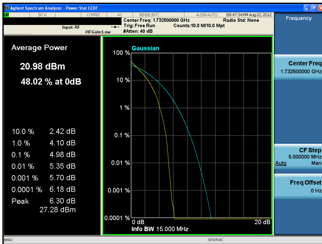
Plot 9-29. PAR Plot (15MHz 16QAM – RB Size 75)
