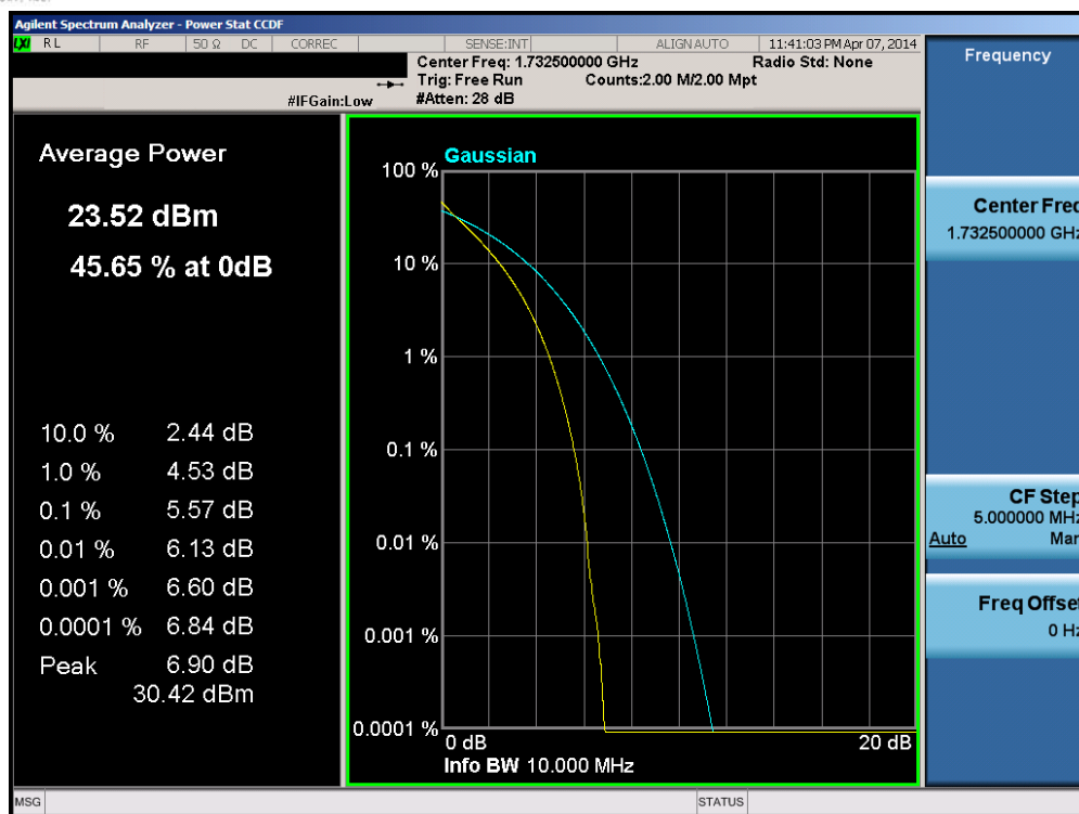
Plot 6-133. PAR Plot (Band 4 – 10.0MHz QPSK – RB Size 50)
