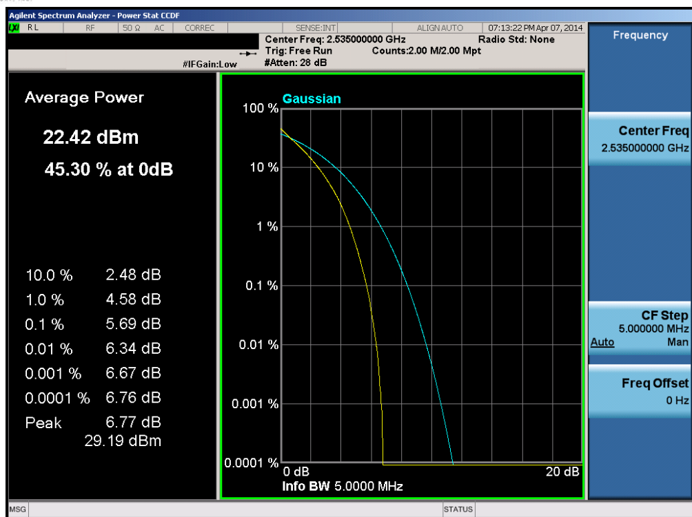
Plot 6-147. PAR Plot (Band 7 – 5.0MHz QPSK – RB Size 25)
