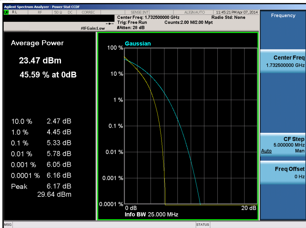
Plot 6-135. PAR Plot (Band 4 – 15.0MHz QPSK – RB Size 75)
