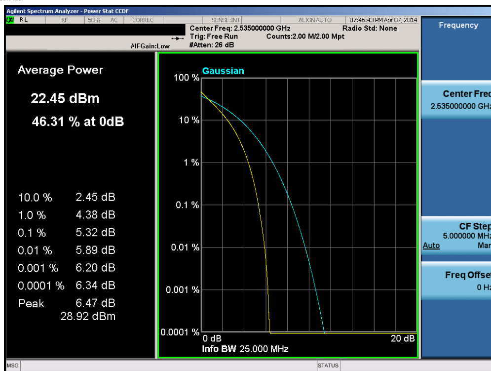
Plot 6-153. PAR Plot (Band 7 – 20.0MHz QPSK – RB Size 100)
