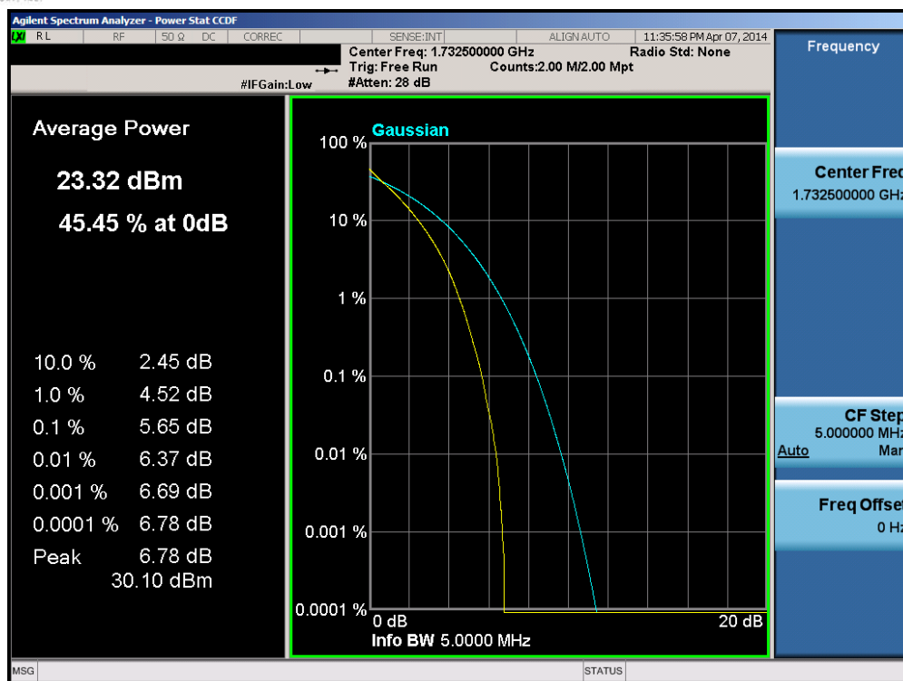
Plot 6-131. PAR Plot (Band 4 – 5.0MHz QPSK – RB Size 25)
