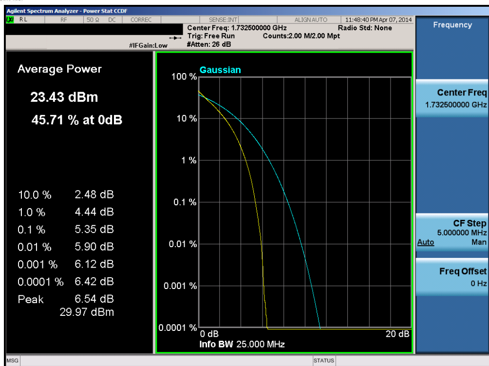
Plot 6-137. PAR Plot (Band 4 – 20.0MHz QPSK – RB Size 100)
