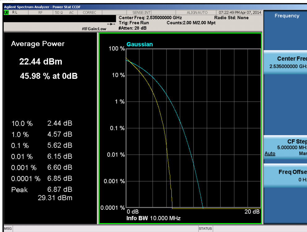
Plot 6-149. PAR Plot (Band 7 – 10.0MHz QPSK – RB Size 50)
