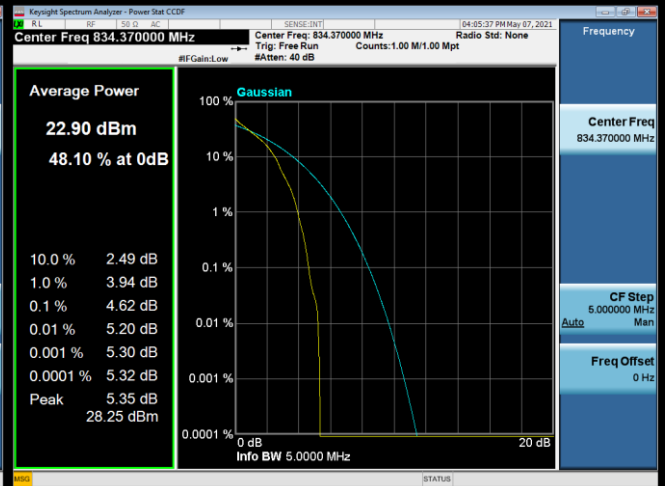
16QAM-20425
