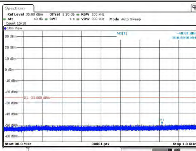
Band41_20MHz_QPSK_39750_1RB#0
