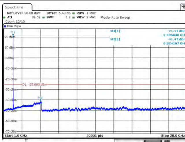
Band41_20MHz_QPSK_39750_1RB#0
