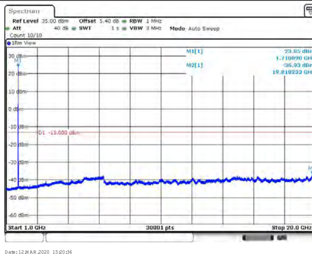
Band4_20MHz_QPSK_20175_1RB#0
