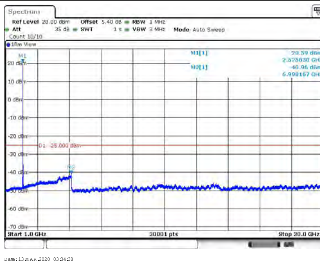
Band7_20MHz_16QAM_21350_1RB#0
