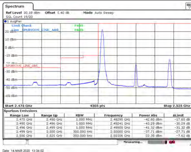
Band7_20MHz_QPSK_20850_100RB#0
