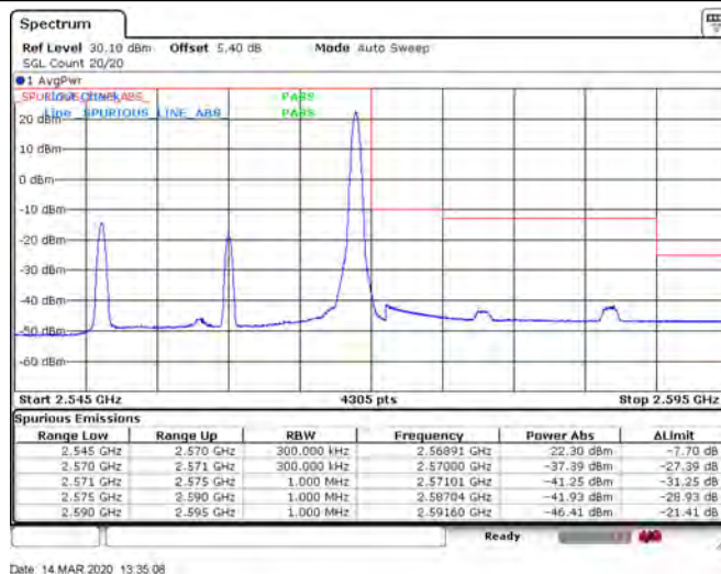
Band7_20MHz_QPSK_21350_100RB#0
