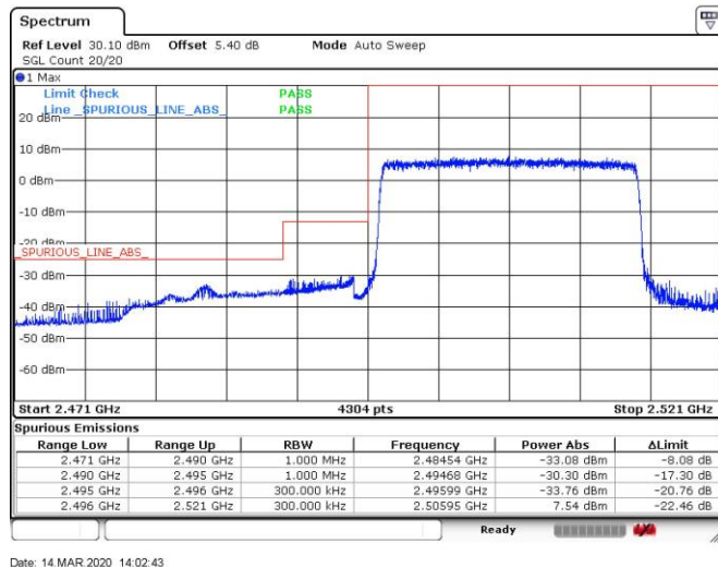
Band41_20MHz_QPSK_41490_1RB#99
