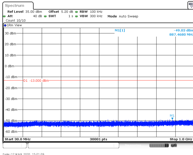
Band4_20MHz_QPSK_20175_1RB#0
