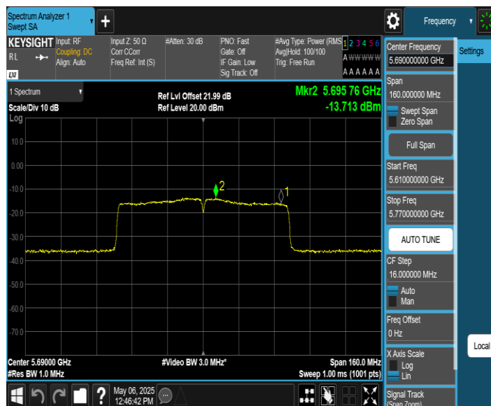
11AC80SISO_Ant1_5690_UNII-3
