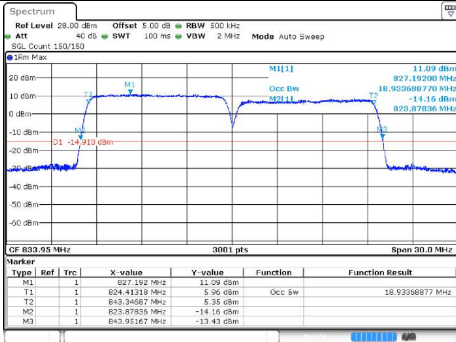
CA 5B 50RB+50RB 64QAM 20450+20549 50RB#0+50RB#0
