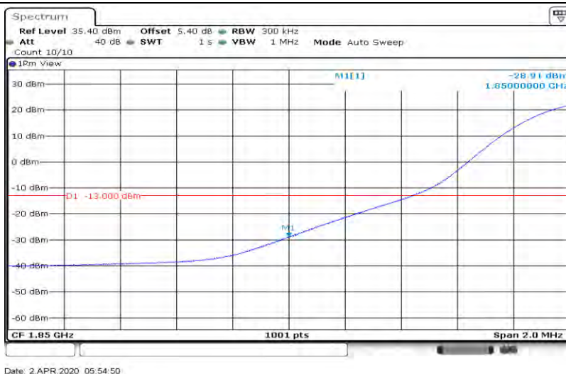
Band2-20MHz-QPSK-18700-100RB#0
